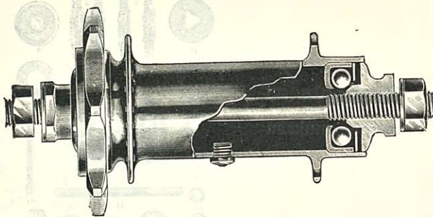
N:o 181. Takapyörän rumpu ketjurattaan kanssa.
