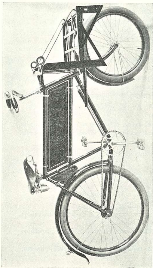
Tavarankuljetuspyörä N:o 12/22.
