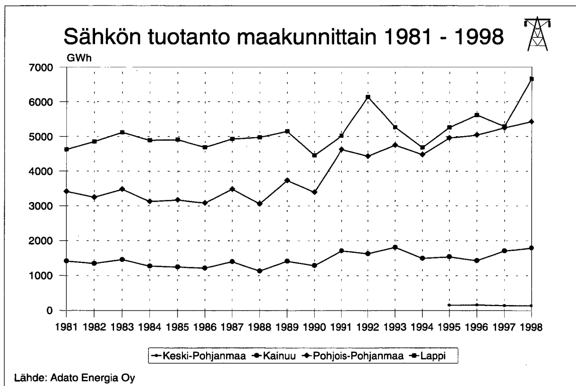
Kuva 109. Sähkön tuotanto maakunnittain 1981 – 1998.
