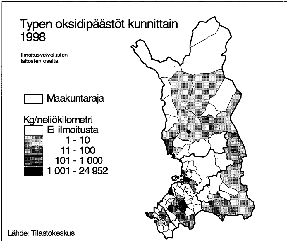
Kuva 119. Typen oksidipäästöt ( \text{No}_x ) kunnittain 1998.
