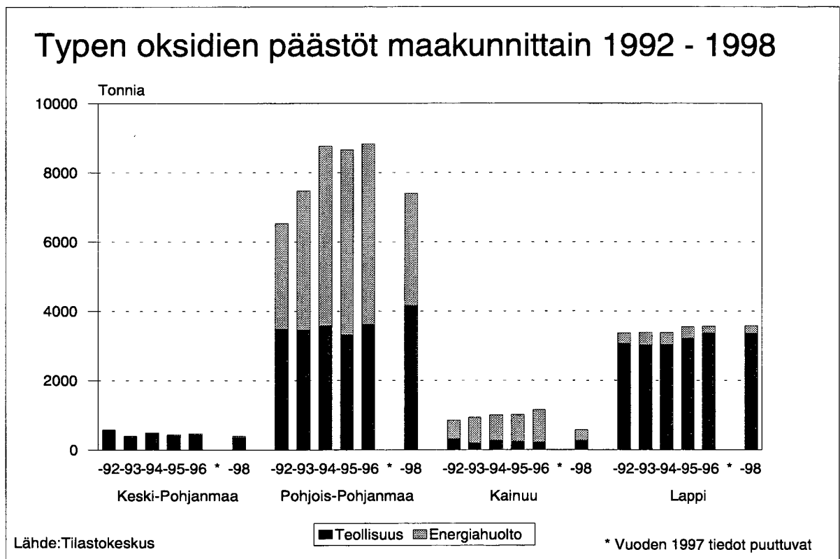
Kuva 116. Typen oksidien päästöt maakunnittain 1992 - 1998.
