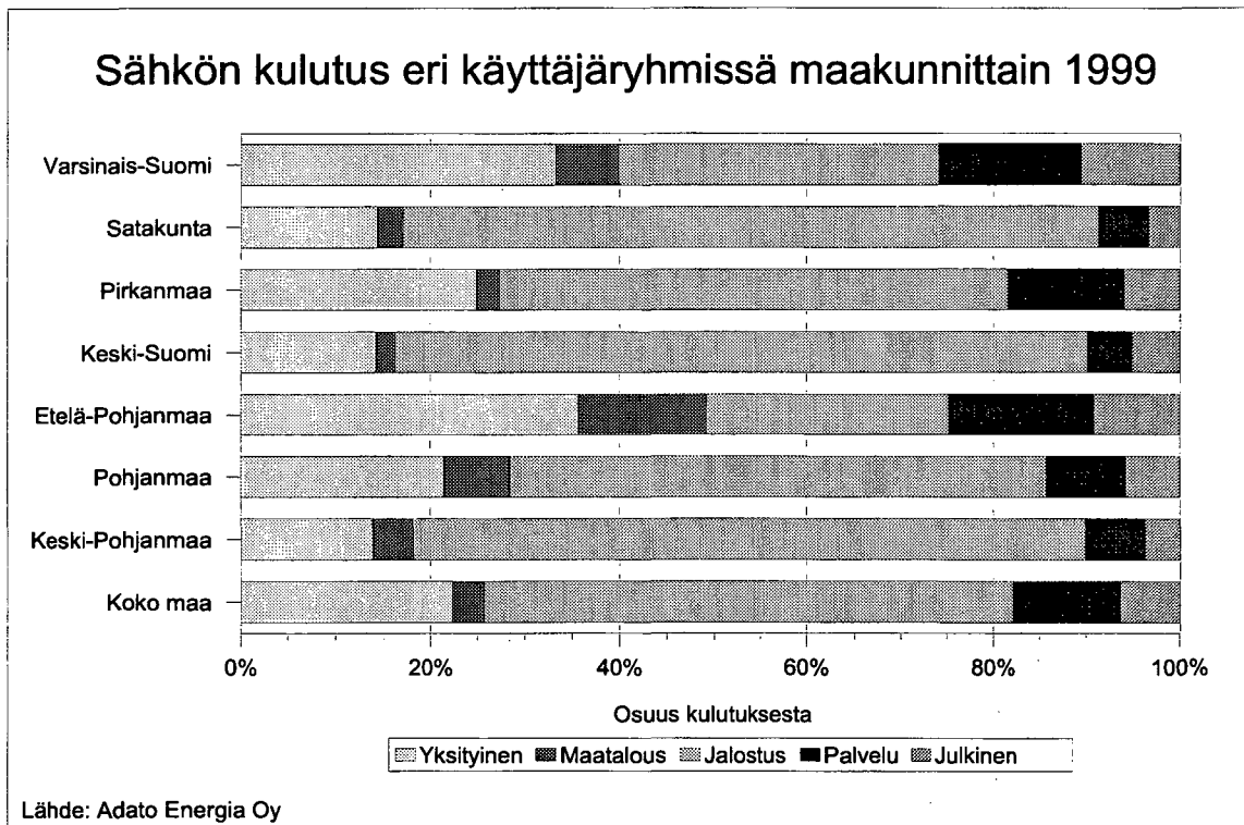
Kuva 107. Sähkön kulutus eri käyttäjäryhmissä maakunnittain 1999.
