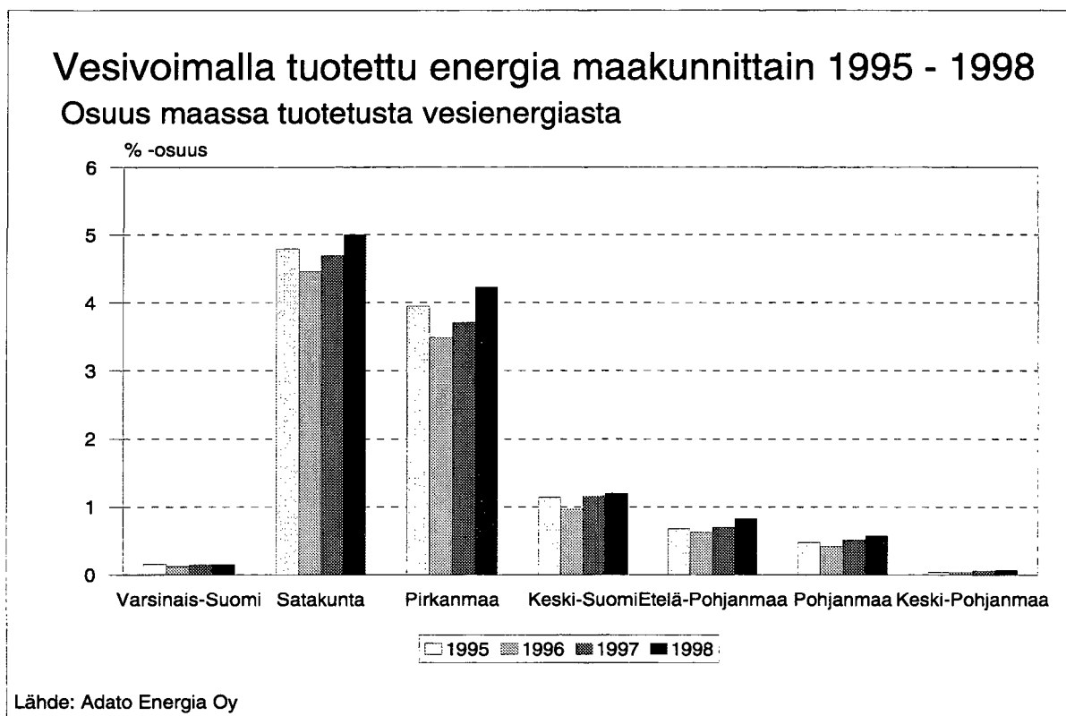
Kuva 107. Vesivoimalla tuotettu energia maakunnittain 1995 – 1998.
