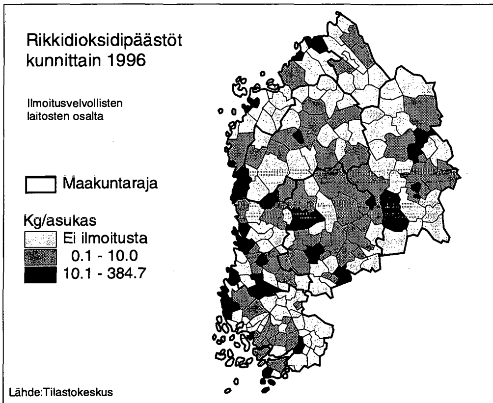
Kuva 120. Rikkidioksidipäästöt ( \text{SO}_2 ) kunnittain 1996.
