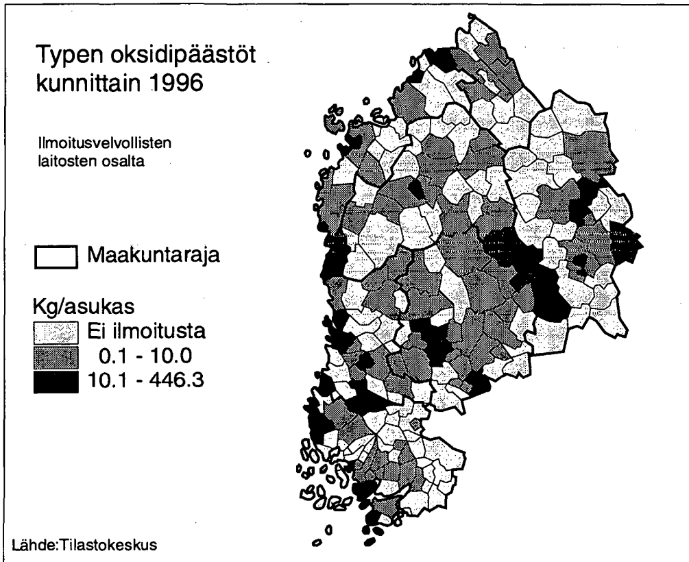
Kuva 119. Typen oksidipäästöt ( \text{No}_x ) kunnittain 1996.
