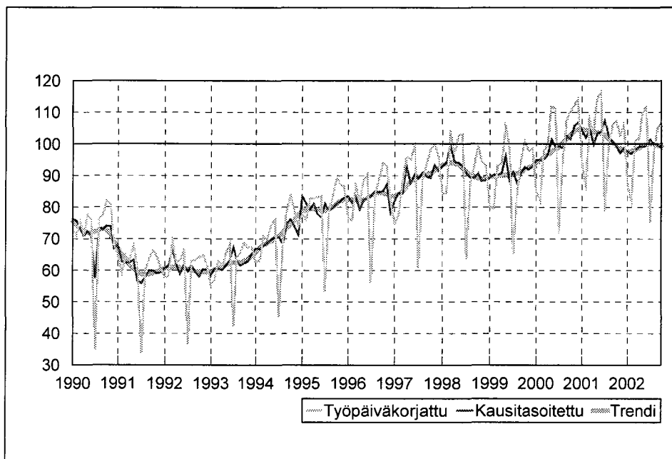
Kuvio 9. Muu metalliteollisuus TOL met -DL, teollisuustuotannon volyyymi-indeksi 1990 – 2002 marraskuu, 2000=100
