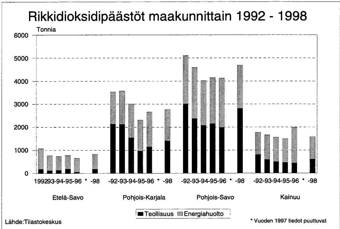
Kuva 117. Rikkidioksidipäästöt maakunnittain 1992 - 1998.
