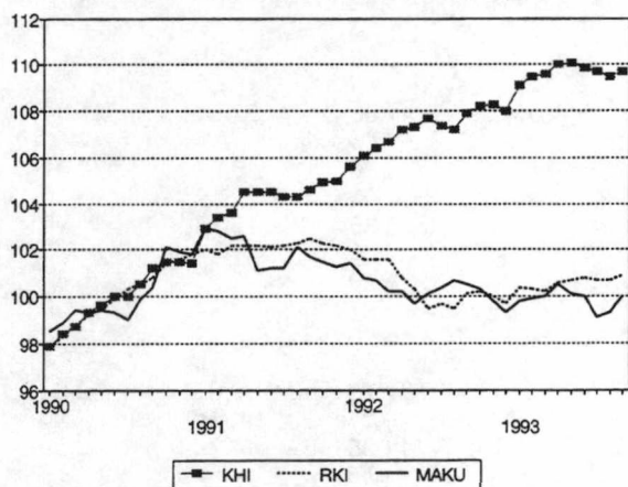
Kuluttajahintaindeksin rakennuskustannusindeksin ja maarakennuskustannusindeksin kehitys
