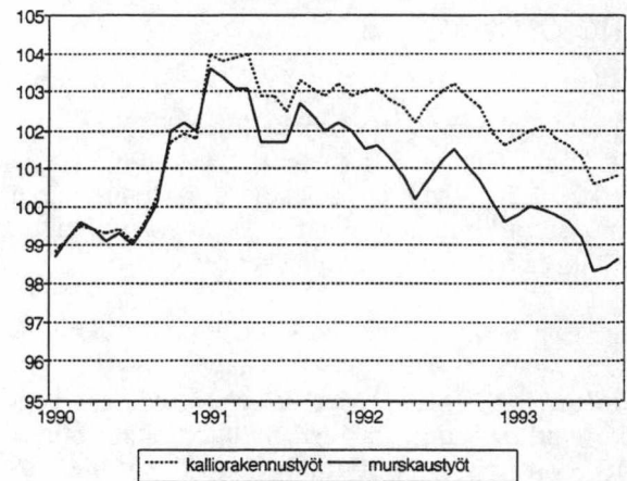
Maarakennuskustannusindeksin työläjien kustannuskehitys
