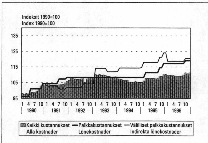
Kuvio 4.1 – Figur 4.1 Kuorma-autoliikenteen kustannusindeksi (tammikuu 1990 – joulukuu 1996) Kostnadsindex för lastbilstrafiken (januari 1990 – december 1996)
