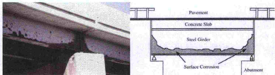
Kuva 14 Teräspalkki- ja betonikansirakenteisen terässillan tyypillinen korroosio (Lee et al. 2006).
