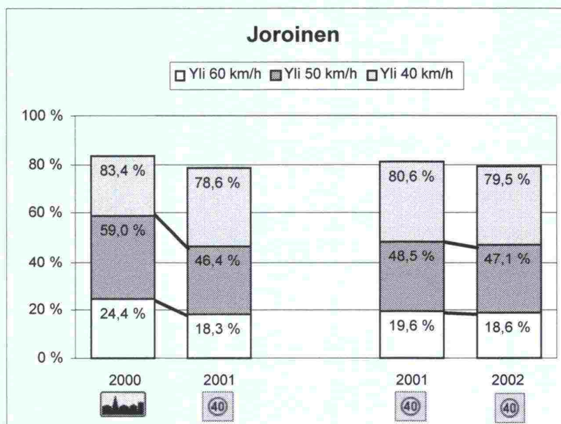
Kuva 6-8. Nopeusrajoituksen alentamisen vaikutus (2000 - 2001) ja heräteraitojen sekä tiemeraintöjen vaikutus (2001 - 2002) eri nopeuden ylittäneiden ajoneuvojen osuuksiin eri mittausvuosina.
