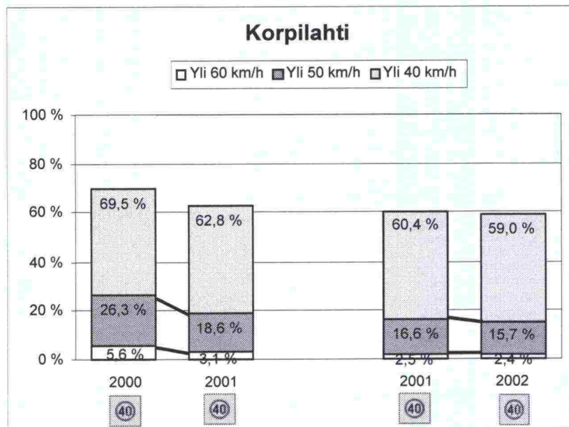
Kuva 6-16. Korpilahdentien saneerauksen vaikutus eri nopeuden ylittäneiden ajoneuvojen osuuksiin eri mittausvuosina.
