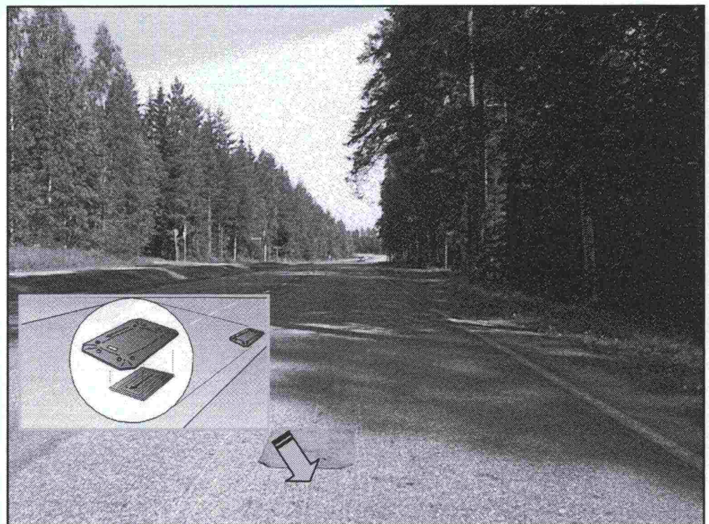
Kuva 3-1. HI-STAR - liikennelaskentalaitte asennettuna tienpintaan Hankasalmella pisteessä 3 (mittaussuunta keskustaan päin). /4.
