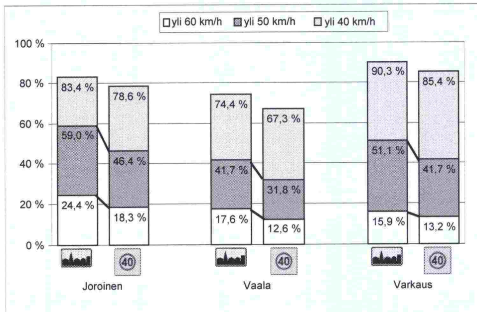
Kuva 6-4. Nopeusrajoituksen alentamisen vaikutus eri nopeuden ylittäneiden ajoneuvojen määrään eri taajamissa. Keskiarvoissa ovat mukana kyseisen taajaman ne pisteet, joista on tulokset molemmilta vuosilta.
