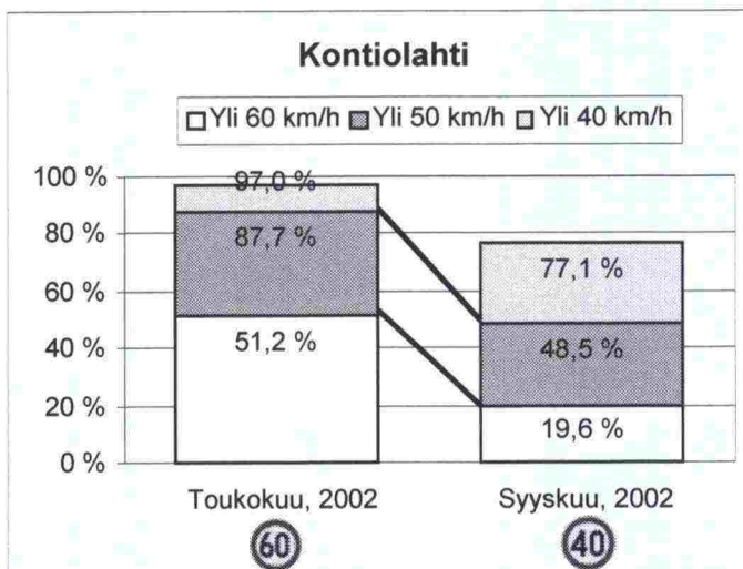
Kuva 6-14. Töyssyn vaikutus (toukokuu 2002 - syyskuu 2002) vaikutus eri nopeuden ylittäneiden ajoneuvojen osuuksiin. Keskiarvoissa ovat mukana pisteet 1-5. Pisteessä 1 oli voimassa syyskuun mittauksen aikana 60 km/h nopeusrajoitus.
