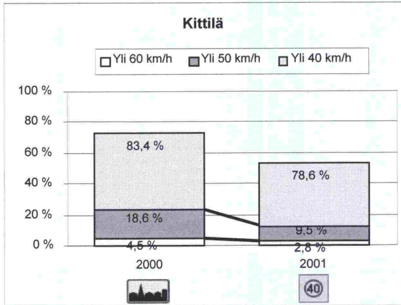
Kuva 6-10. Nopeusrajoituksen alentamisen ja tiemerkitöjen vaikutus eri nopeuden ylittäneiden ajoneuvojen osuuksiin eri mittausvuosina.
