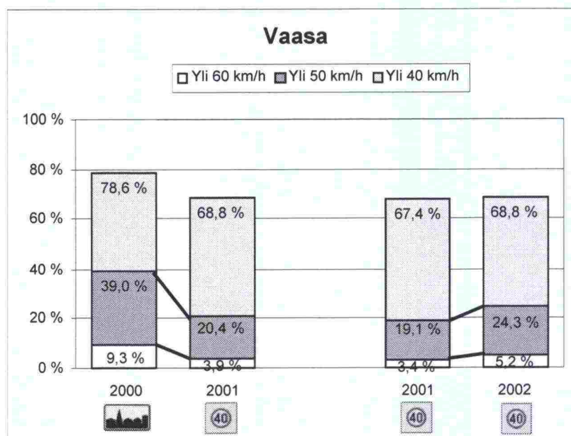
Kuva 6-6. Nopeusrajoituksen alentamisen vaikutus eri nopeuden ylittäneiden ajoneuvojen osuuksiin eri mittausvuosina.
