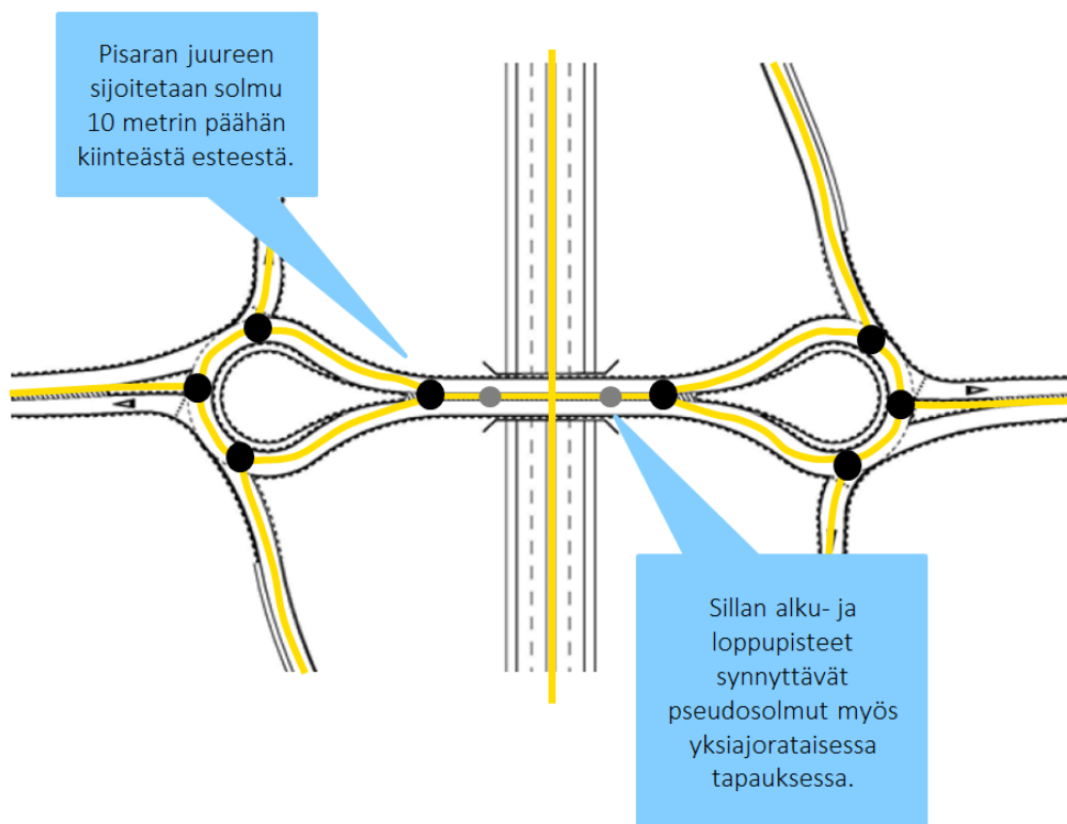
Kuva 18. Pisaraliittymä, esimerkki samasta kohdasta yhden ajoradan yhdistämänä.
