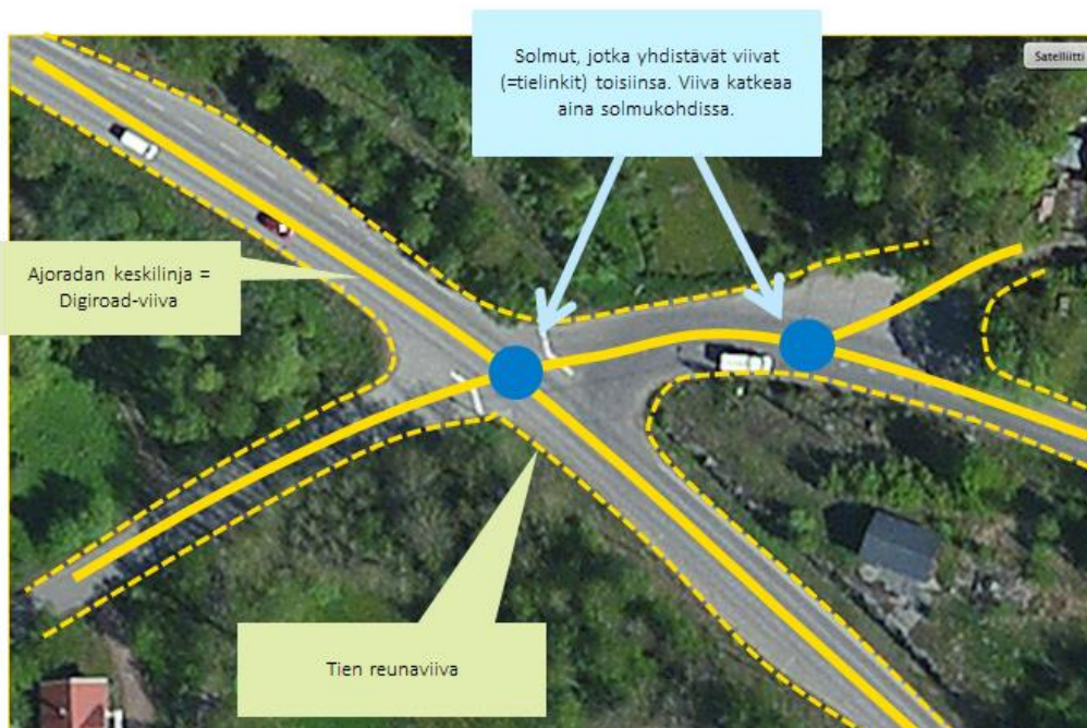
Kuva 1. Perusperiaate linkkien katkeamiskohdista.
