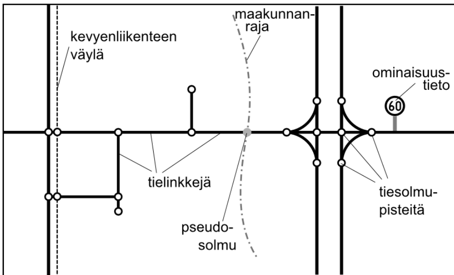
Kuva 1. Tielinkki ja tiesolmupisteet (kuva JHS 188)
