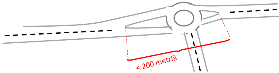
Kuva 16d. Kiertoliittymä alle 200 metrisen kaksiajorataisen osuuden välissä kuvataan kalapyrstöllä, jos yksittäinen fyysinen jakaja täyttää ”kalapyrstöille asetetut minimimitat (liikenteenjakaajan pituus on yli 25 m ja jakajan leveys yli 10 m tai liikenteenjakaajien ulkoreunojen välinen etäisyys on yli 10 m ja pituus yli 25 m.). Katso haaraumia tarkemmin koskevat säännöt ohjeen kohdasta 3.4.9 Haaraumat. Jos haaraumasäännöt eivät täyty, kuvataan ajotiet yksiajorataisena geometriana.
