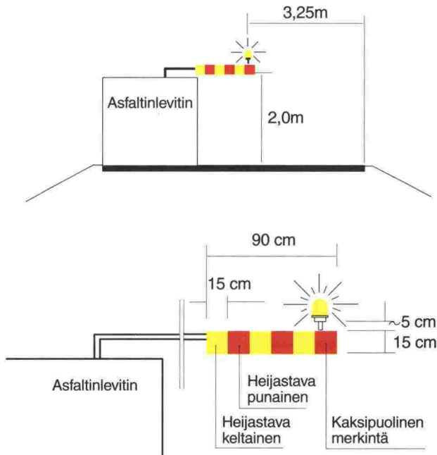
Asfaltinlevittimen varoitusmerkintä
