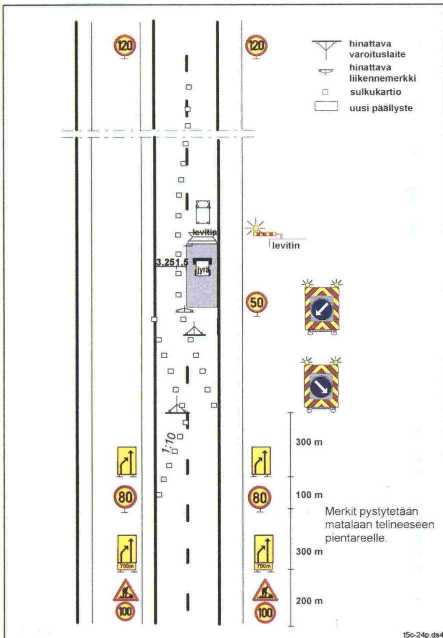
Moottoritie, liikenne samalla ajoradalla
