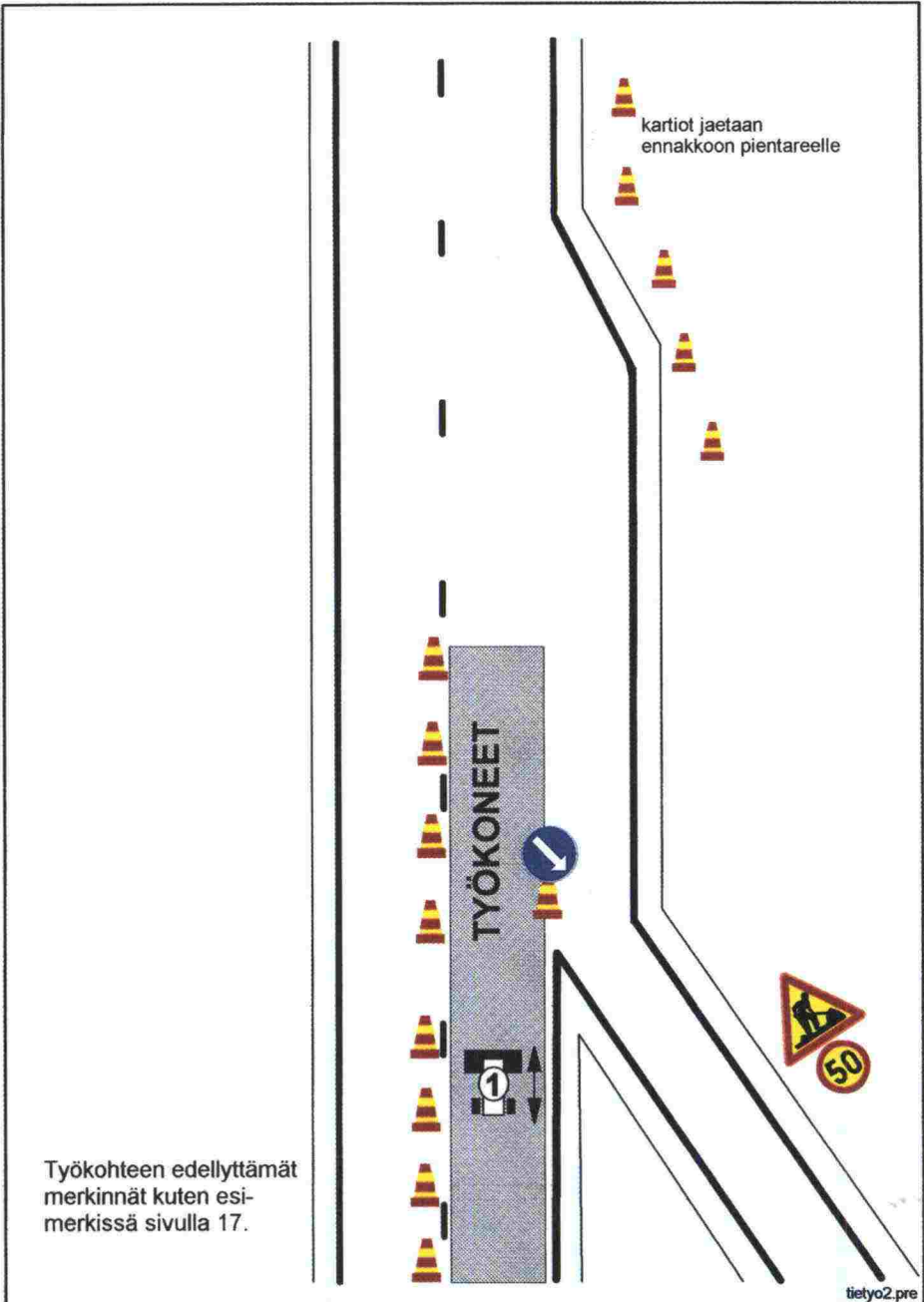
Moottoritie, liittyminen rampilta, vaihe 1
