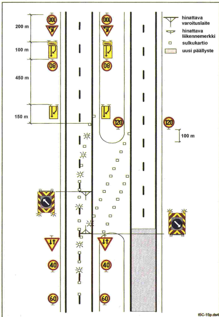
Moottoritie, liikenne ohjattu kokonaan toiselle ajoradalle (työkohde päättyy)
