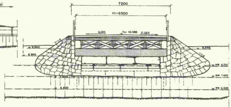
B-B, 1:50
