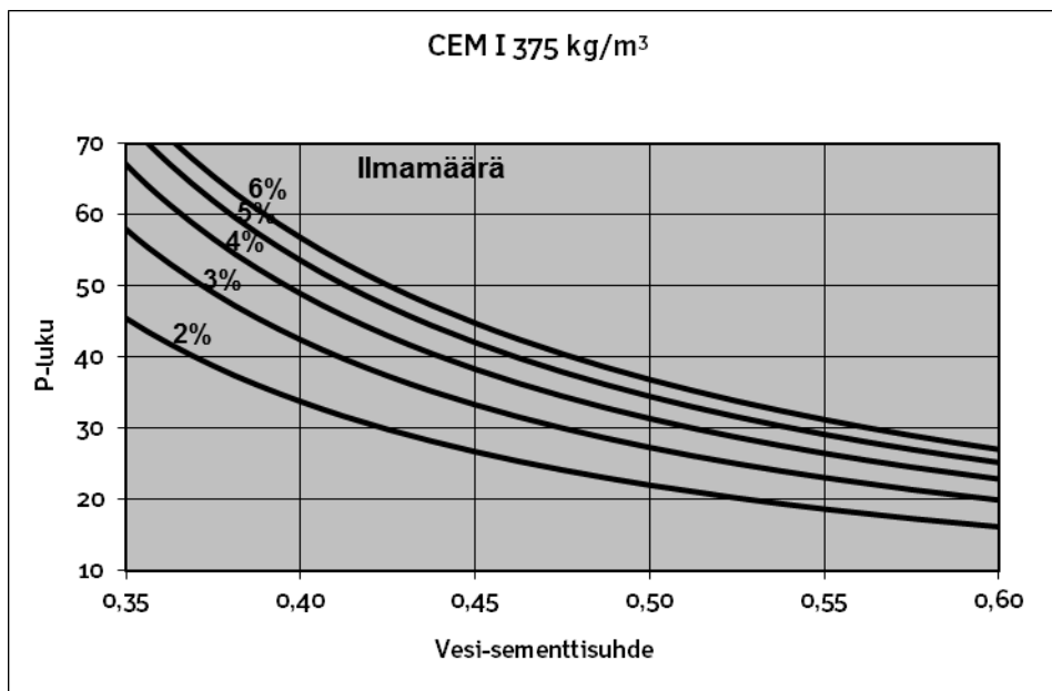
Kuva 2. Esimerkki kaavalla 1 lasketun P-luvun riippuvuudesta vesi-sementtisuhteesta ja ilmamäärästä sementtitaadulla CEM I sementtimäärän ollessa 375 kg/m^3 . Jälkihoitoaika 7 vuorokautta.
