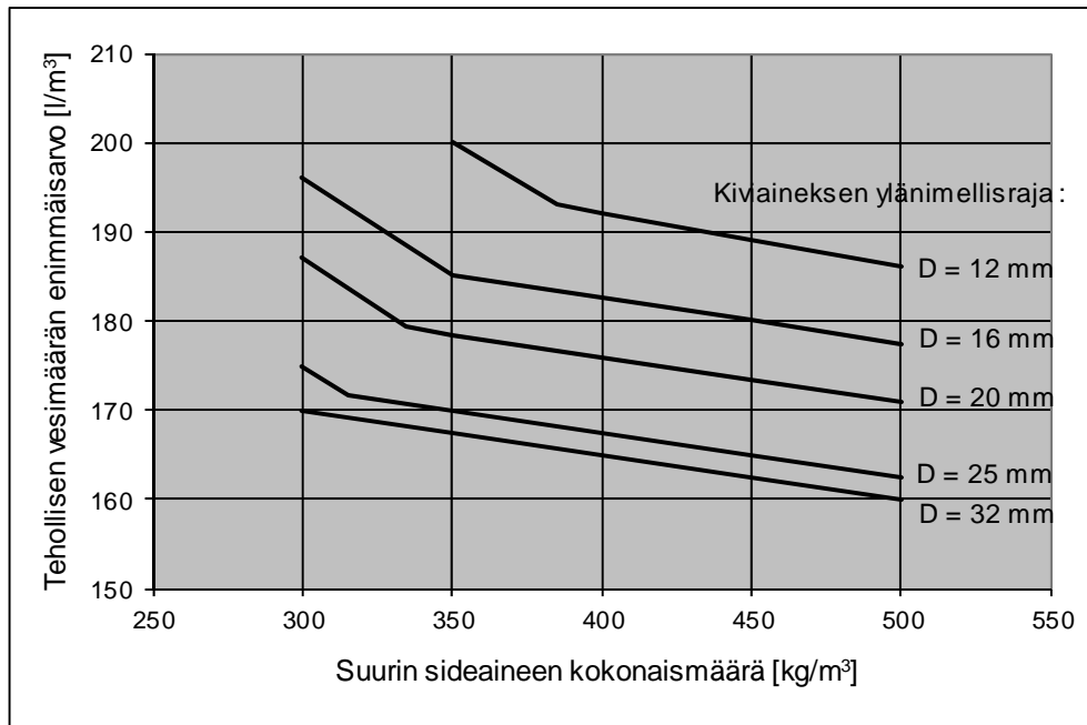
Kuva 1 Suhteituksen suurimman tehollisen vesimäärän ja sideaineen kokonaismäärän välinen riippuvuus, kun kiviaineuksen ylämellisrajat ovat 32, 25, 20, 16 ja 12 mm.
