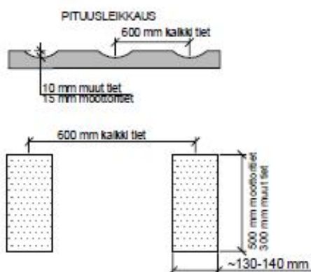
Kuva 17 Jyrsintätavat
