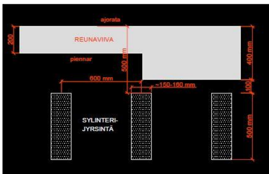
Kuva 18 Sylinterijyrsinnän mitoitusohje
