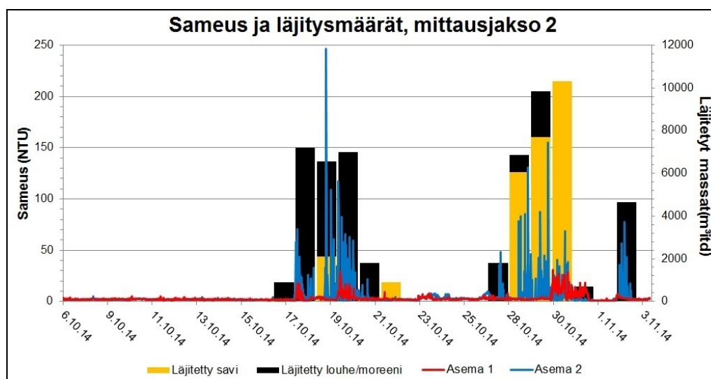
Kuva 27. Jatkuvatoimisten sameusmittausten tulokset sekä läjitysalueelle D läjitetyt massat toisen mittausjakson aikana. Asema 1 sijaitsee läjitysalueen D eteläpuolella ja asema 2 pohjoispuolella. Läjitetyt massat on ilmoitettu yksikössä m 3 /d, joka vastaa proomukuutiota. Läjitetyissä massoissa on eroteltu savi (keltainen väri) sekä louhe/moreeni (musta väri).
