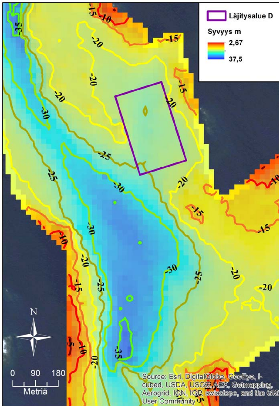
Kuva 11. Pohjan topografia läjitysalueen D läheisyydessä. Pohjan syvyys on kuvattu korkeuskäyrillä ja väreillä siten, että punaiset alueet ovat korkeimpia ja tummansiniset syvimpiä.
