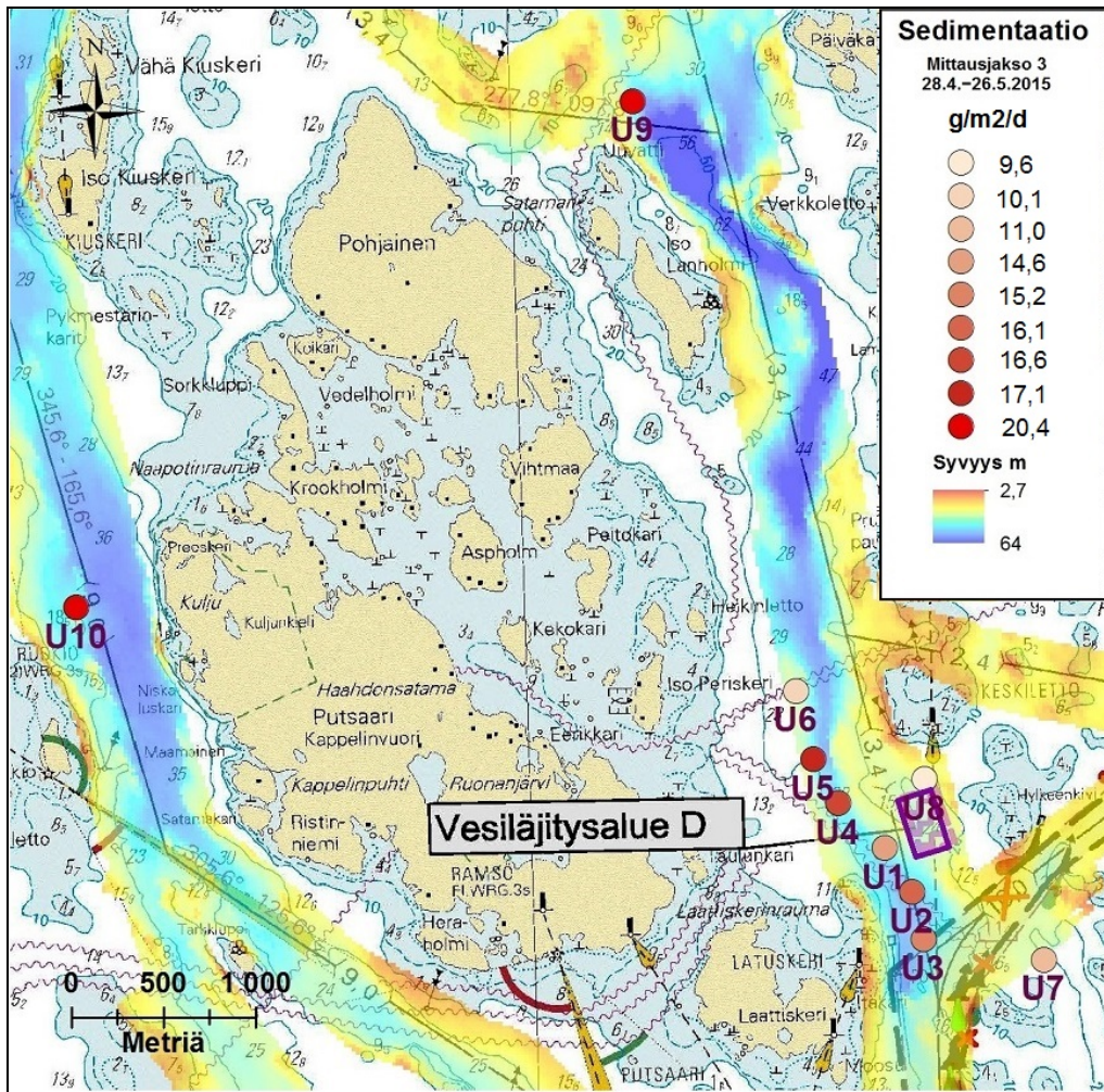
Kuva 35. Sedimentaation määrä keskimäärin vuorokaudessa neliometriä kohden kolmannen mittausjakson aikana. Punaisen värin intensiivisyys kuvaa kertyneen sedimentin määrää näytepisteellä. Pohjakarttana on merikartta, jonka päälle on asetettu alueen merenpohjan topografinen malli.
