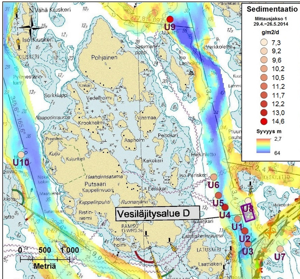
Kuva 33. Sedimentaation määrä keskimäärin vuorokaudessa neliometriä kohden ensimmäisen mittausjakson aikana. Punaisen värin intensiivisyys kuvaa kertyneen sedimentin määrää näytepisteellä. Pohjakarttana on merikartta, jonka päälle on asetettu alueen merenpohjan topografinen malli.
