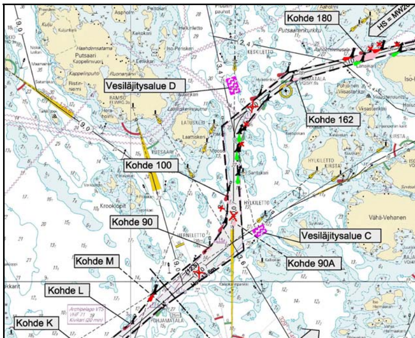
Kuva 5. Ote Uudenkaupungin 12,5 m väylän rakennussuunnitelman yleiskartasta. Kuvassa näkyvät lilalla viivoituksella merkityt läjitysalueet C ja D sekä niiden lähistön ruoppauskohteet vaaleanpunaisina alueina.
