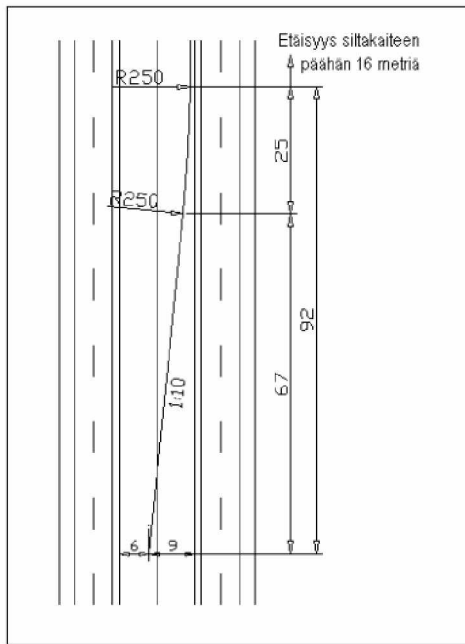
Kuva 1. Kaide keskialueella alikulkusilla kohdalla. Kaide käännetään keskialueelle viistoudessa 1:10.
