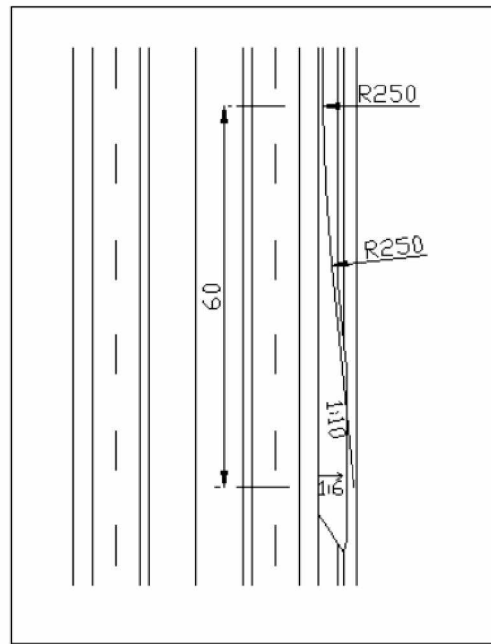
Kuva 2. Kaiteen pään kääntäminen ulkoluiskaan
