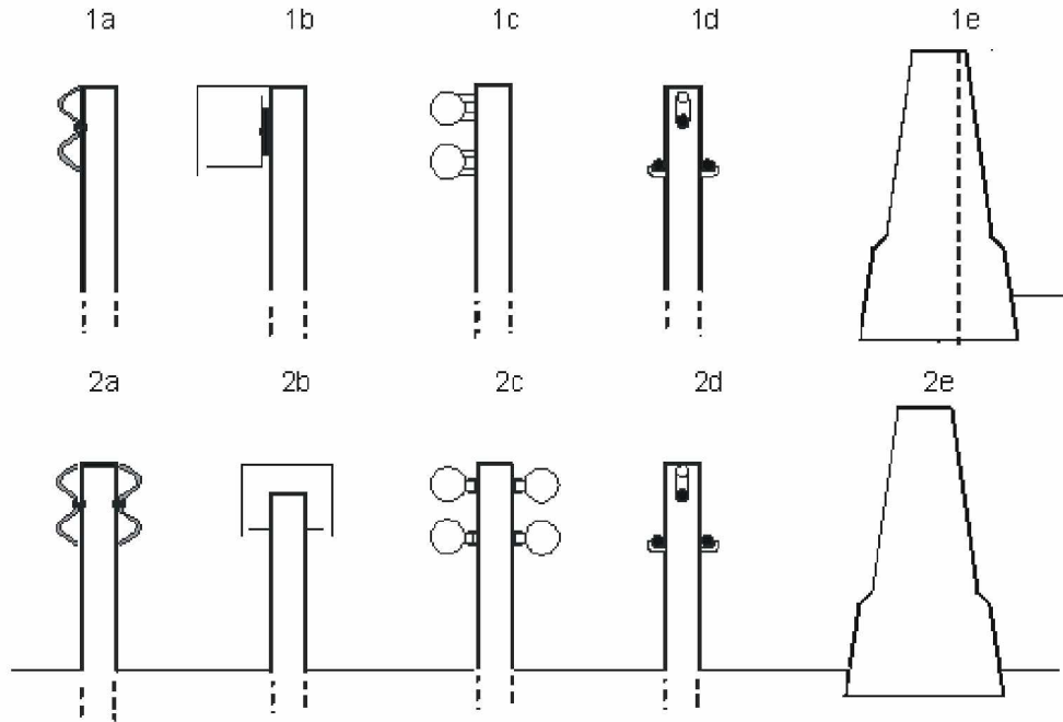
Kuva 9. Kaidetyypit.
