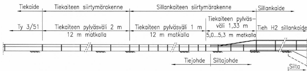
Kuva 6. Esimerkkikuva teräskaiteen liittymisestä sillan kaiteeseen.
