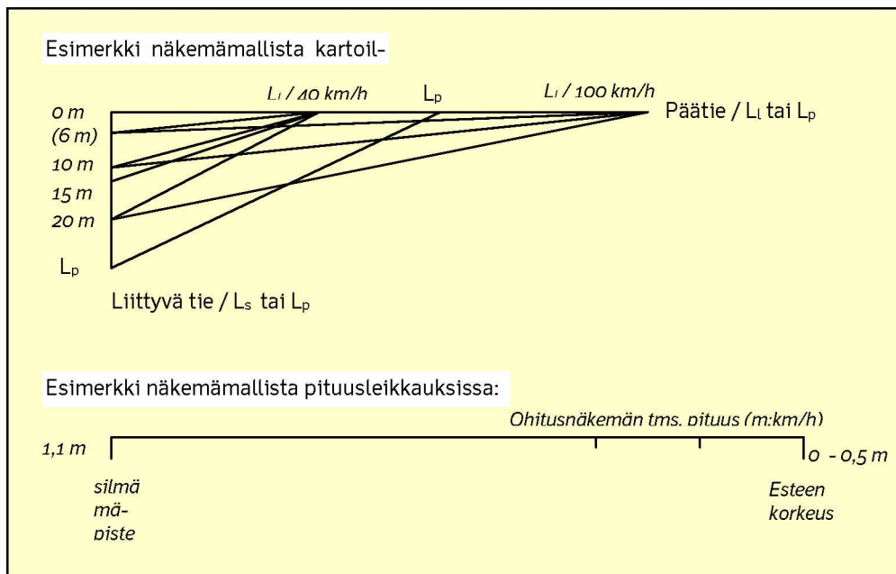
Kuva 6: Esimerkkikuvia näkemämittaustmallin periaatteesta kartalla ja pituusleikkauksessa. Lyhenteet viittaavat ohjeeseen yleisten teiden näkemäalueista.
