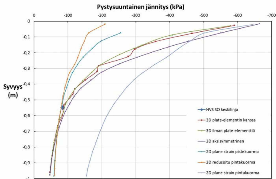
Kuva 66. Mallinnetut ja mitatut pystysuuntaiset jännitykset.
