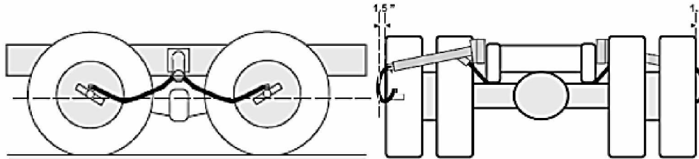
Kuva 14. Säädettävän rengaspainejärjestelmän kytkennät renkaisiin. (TPC International 2013, s. 49, 50)
