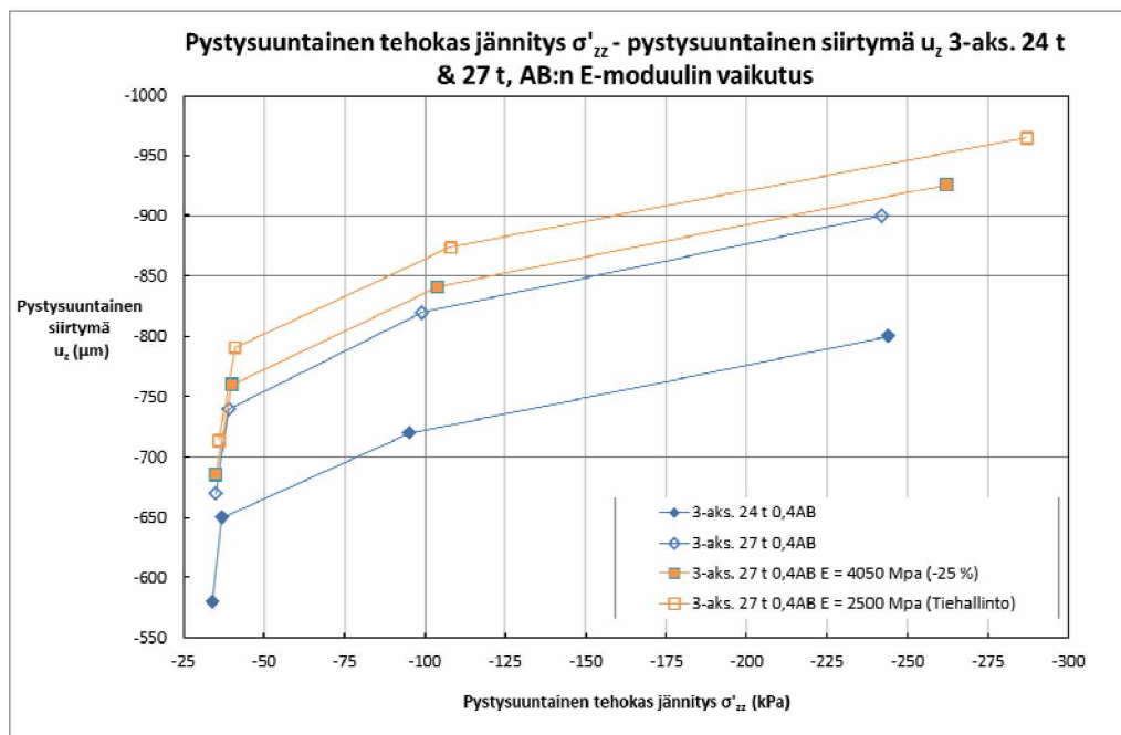
Kuva 85. Pystysuuntainen siirtymä pystysuuntaisen tehokkaan jännityksen funktiona 0,4AB-rakenteen sitomattomien kerrosten keskipisteissä sekä 100 mm syvyydellä pohjamaassa 3-akselisten teliin tapauksissa – AB:n kimmomoduulin vaikutus.
