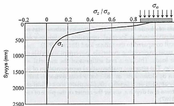
Kuva 47. Jännitys jakauma homogeenisessä puoliavaruudessa ( \nu=0,35 ), jota kuormittaa halkaisijaltaan 300 mm levy. (Mukaiituna Doré & Zubeck 2009, s. 40)
