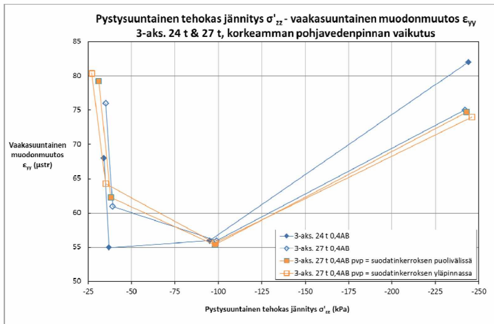
Kuva 90. Vaakasuuntainen muodonmuutos pystysuuntaisen tehokkaan jännityksen funktiona 0,4AB-rakenteen sitomattomien kerrosten keskipisteissä sekä 100 mm syvyydellä pohjamaassa 3-akselisten telien tapauksissa – korkeamman pohjavedenpinnan vaikutus.
