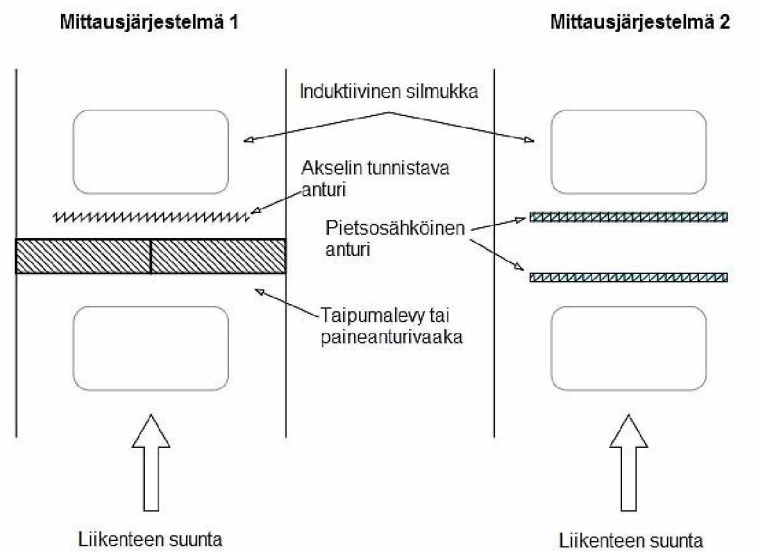
Kuva 43. Kaksi tyypillistä WIM-mittausjärjestelyä: taipumalevyyn tai paineanturi-vaakaan perustuva järjestelmä sekä pietsosähköisiin antureihin perustuva järjestelmä. (Mukaiituna Lu ym. 2002, s. 26)
