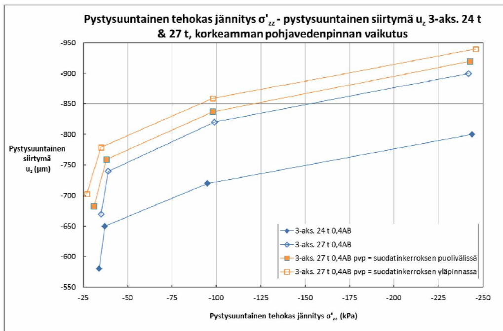
Kuva 89. Pystysuuntainen siirtymä pystysuuntaisen tehokkaan jännityksen funktiona 0,4AB-rakenteen sitomattomien kerrosten keskipisteissä sekä 100 mm syvyydellä pohjamaassa 3-akselisten telien tapauksissa – korkeamman pohjavedenpinnan vaikutus.
