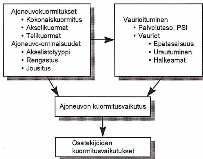
Kuva 40. Ajoneuvojen kuormitusvaikutusten selvittäminen koetiekokeella. (Ehrola 1996, s. 49)
