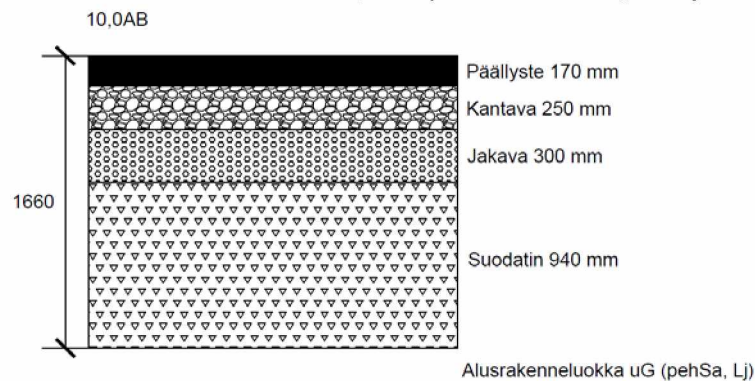
Kuva 63. Tarkasteltava tierakenne 10,0AB. (Tiehallinto 2004, s. 66)
