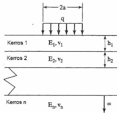
Kuva 48. Ympyränmuotoisen tasaisen kuorman kuormittama monikerrosrakenne. (Huang 2012, s. 57)
