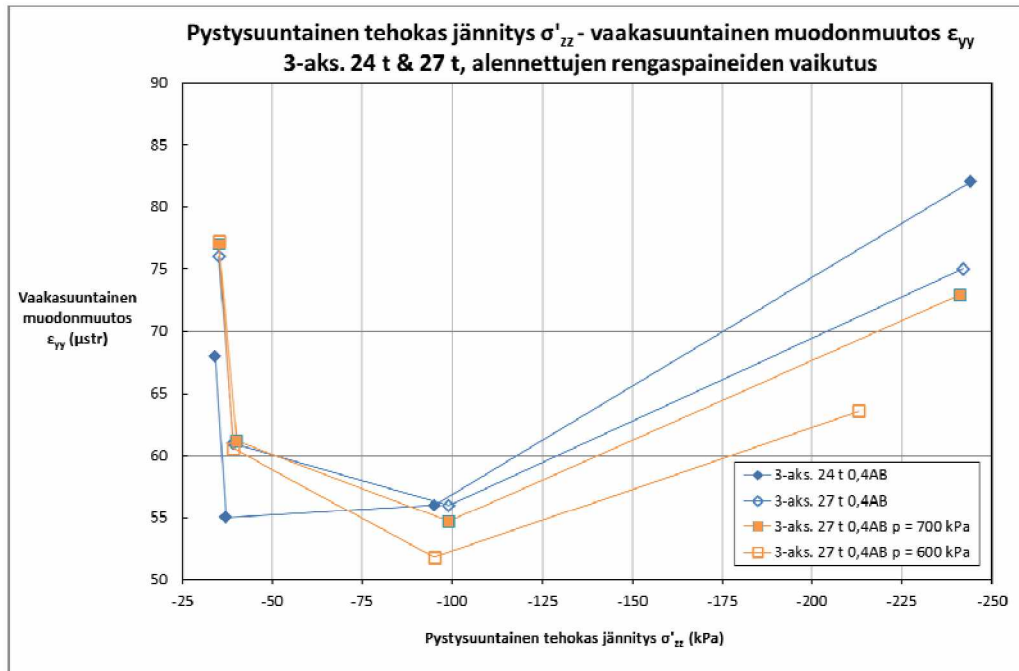
Kuva 84. Vaakasuuntainen muodonmuutos pystysuuntaisen tehokkaan jännityksen funktiona 0,4AB-rakenteen sitomattomien kerrosten keskipisteissä sekä 100 mm syvyydellä pohjamaassa 3-akselisten telien tapauksissa – alennettujen rengaspaineiden vaikutus.
