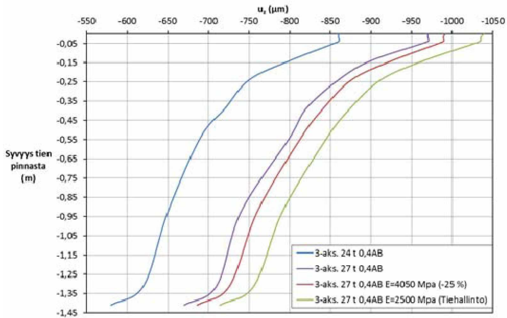
Pystysuuntainen hetkellinen siirtymä u_z , 3-aks., heikkomman AB:n vaikutus
