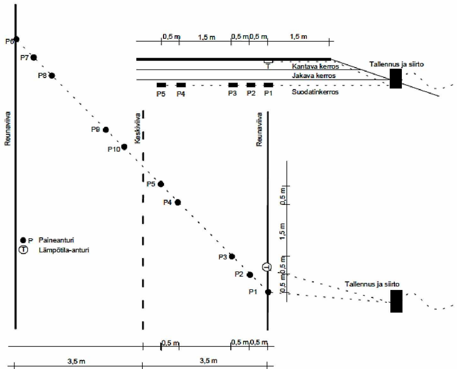
Kuva 44. Esimerkki paineantureihin perustuvasta mittausjärjestelmästä 7 metriä leveällä ajoradalla. (Savolainen ym. 2001b, s. 62)
