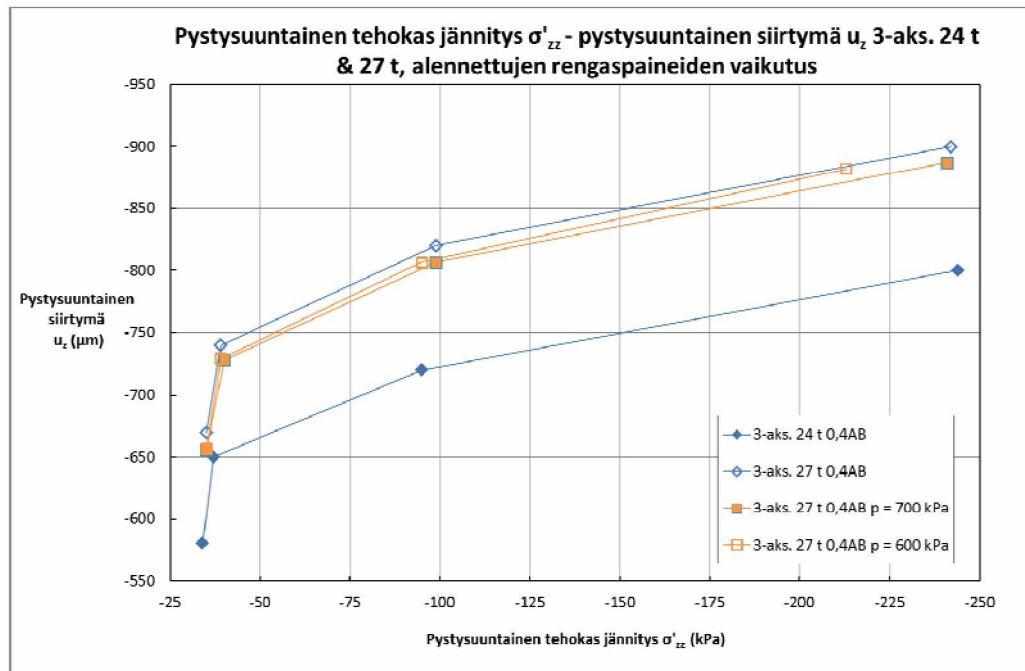
Kuva 83. Pystysuuntainen siirtymä pystysuuntaisen tehokkaan jännityksen funktiona 0,4AB-rakenteen sitomattomien kerrosten keskipisteissä sekä 100 mm syvyydellä pohjamaassa 3-akselisten telien tapauksissa – alennettujen rengaspaineiden vaikutus.
