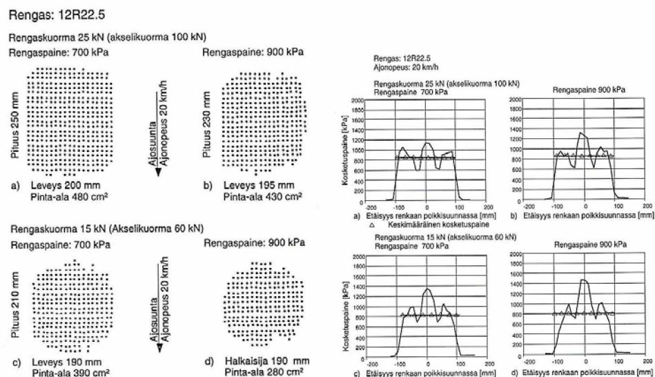
Kuva 12. Kuorma-auton paripyörärenkaan 12R22,5 kosketuskuvion muoto ja koko sekä kosketuspaineen jakauma renkaan poikkisuunnassa erilaisilla rengaskuormilla ja -paineilla. (Ehrola 1996, s. 43, 45)
