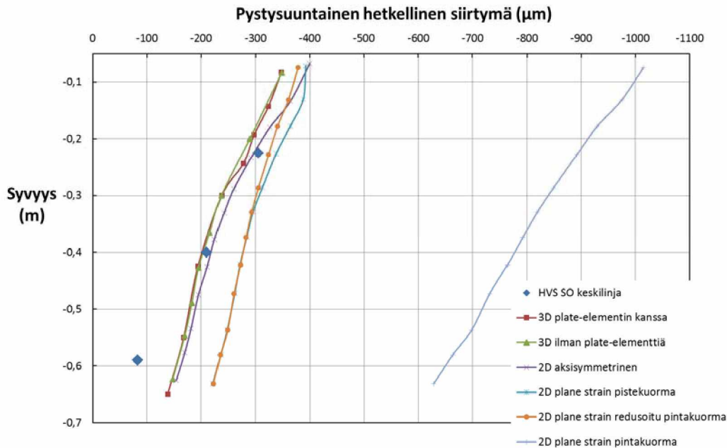
Kuva 65. Mallinnetut ja mitatut pystysuuntaiset hetkelliset siirtymät.
