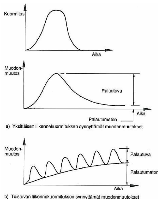
Kuva 28. Tierakenteen ja sen materiaalien muodonmuutoskäyttäytymisen periaate. (Ehrola 1996, s. 171)
