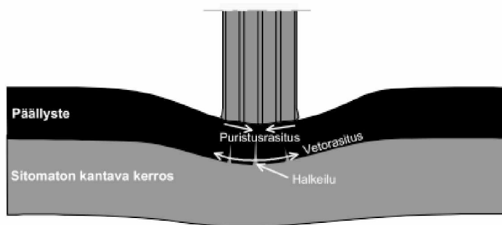
Kuva 21. Liikennekuorman aiheuttamat rasitukset päällysteeseen ja niiden aikaansaama halkeilu. (Belt ym. 2000, s. 41)
