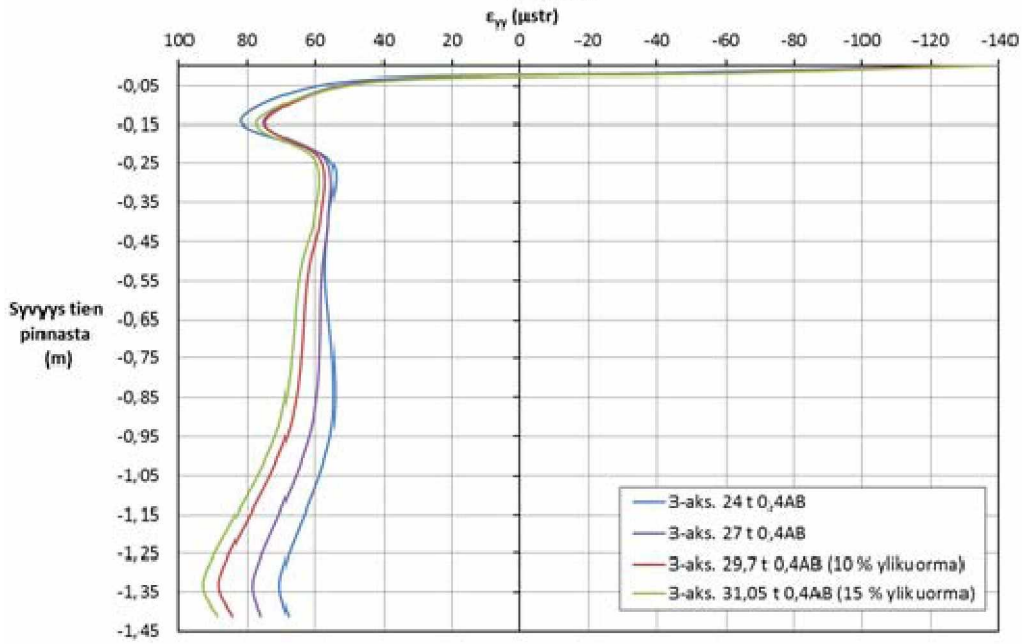
Vaakasuuntainen suhteellinen muodonmuutos \epsilon_{yy} , 3-aks., ylikuorman vaikutus
