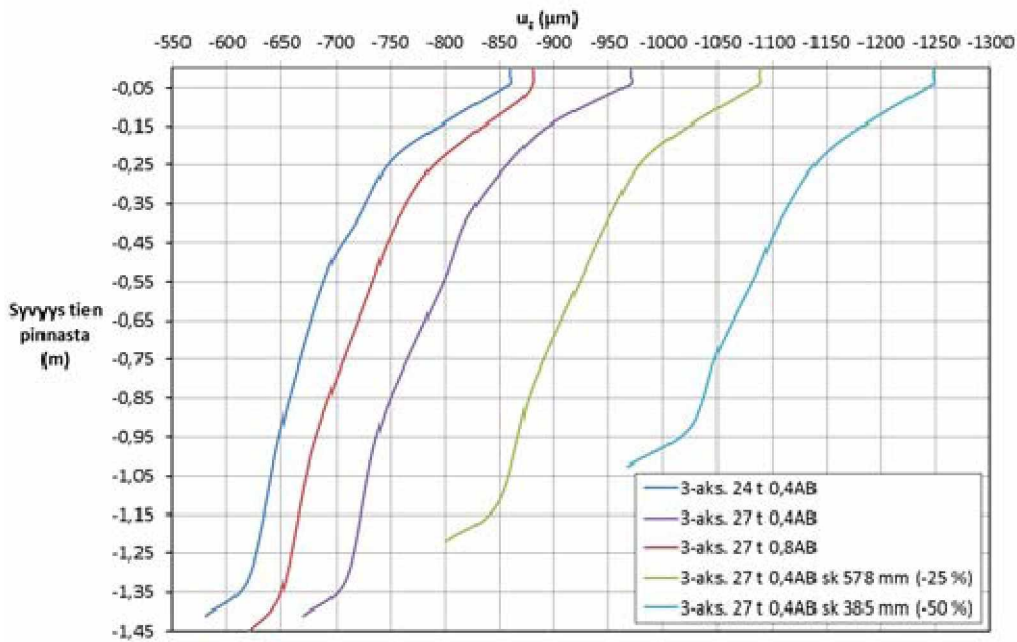
Pystysuuntainen hetkellinen siirtymä u_z , 3-aks., paksumman AB:n ja ohuemman suodatinkerroksen vaikutus
