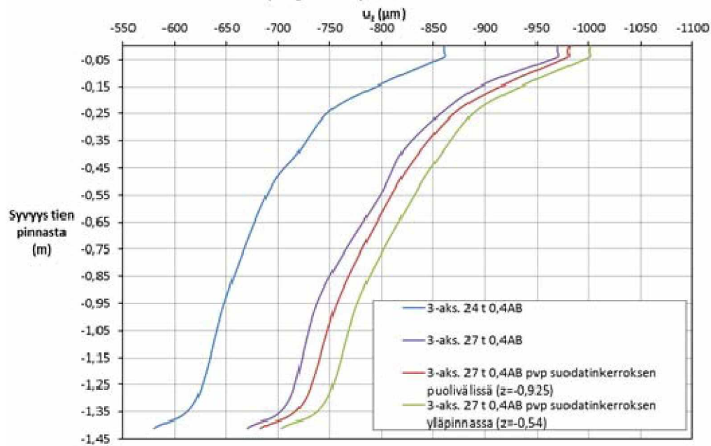
Pystysuuntainen hetkellinen siirtymä u_z , 3-aks., korkeamman pohjavedenpinnan vaikutus
