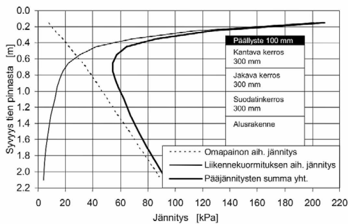
Kuva 34. Pääjännitysten summan muodostumisen periaate. (Belt ym. 2000, s. 33)
