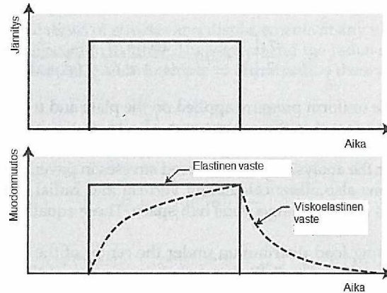
Kuva 45. Elastinen ja viskoelastinen jännitys-muodonmuutuskäyttäytyminen. (Mukailtuna Doré & Zubeck 2009, s. 39)
