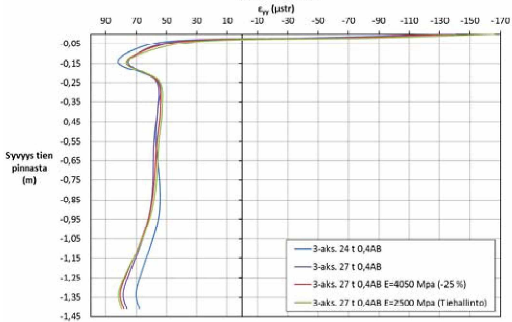
Vaakasuuntainen suhteellinen muodonmuutos \epsilon_{yy} , 3-aks., heikkomman AB:n vaikutus
