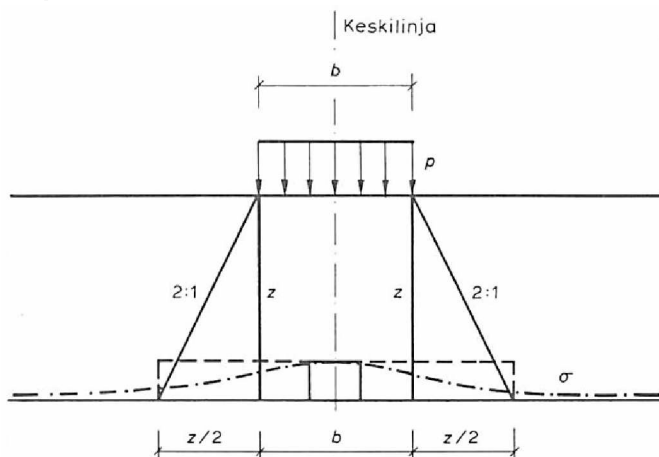
Kuva 50. Pystysuuntaisen jännityksen määrittäminen pitkänomaisen perustuksen keskilinjalla 2:1-menetelmällä. (RIL 1985, s. 346)
