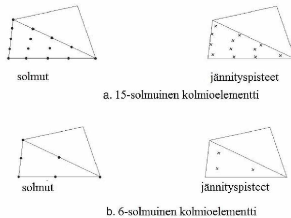
Kuva 57. Elementtityypit Plaxis 2D:ssä. (Brinkgreve ym. 2011c, s. 17)
