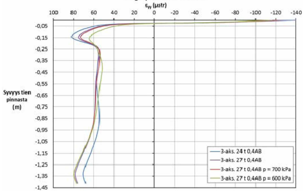
Vaakasuuntainen suhteellinen muodonmuutos \epsilon_{yy} , 3-aks., alennettujen rengaspaineiden vaikutus
