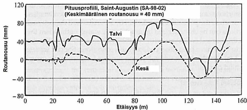
Kuva 25. Kesällä ja talvella mitatut moreenille perustetun tierakenteen pituusprofiilit. (Mukaiituna Doré & Zubeck 2009, s. 89)
