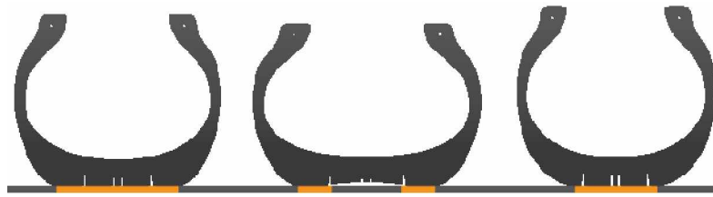
Kuva 13. Rengaspaineen vaikutus renkaan muotoon ja kosketuspinta-alaan: vasemmalla oikea rengaspaine, keskellä liian pieni rengaspaine ja oikealla liian suuri rengaspaine. (Tyreright 2012)
