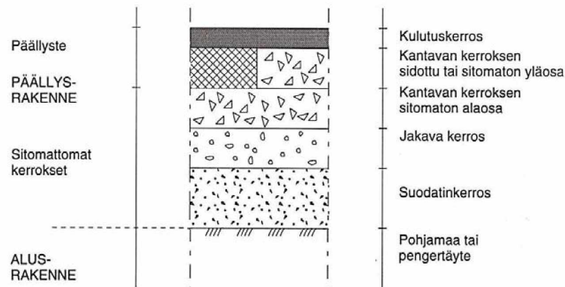
Kuva 17. Päälystetyn tierakenteen tyypilliset rakennekerrokset. (Ehrola 1996, s. 138)
