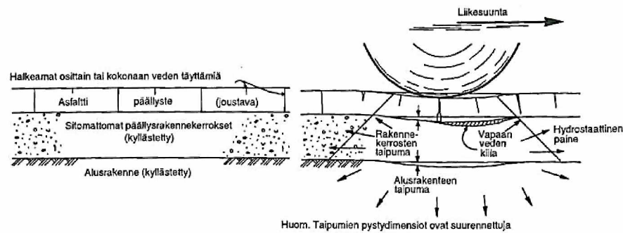
Kuormittamaton joustava tierakenne Kuormitettu joustava päällysrakenne
