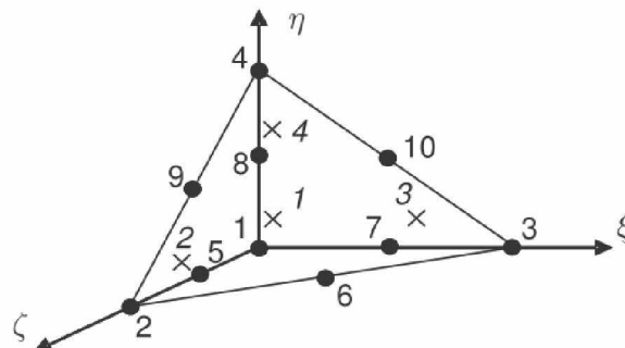
Kuva 58. Plaxis 3D:n 10-solmuinen elementti. (Brinkgreve ym. 2012, s. 148)
