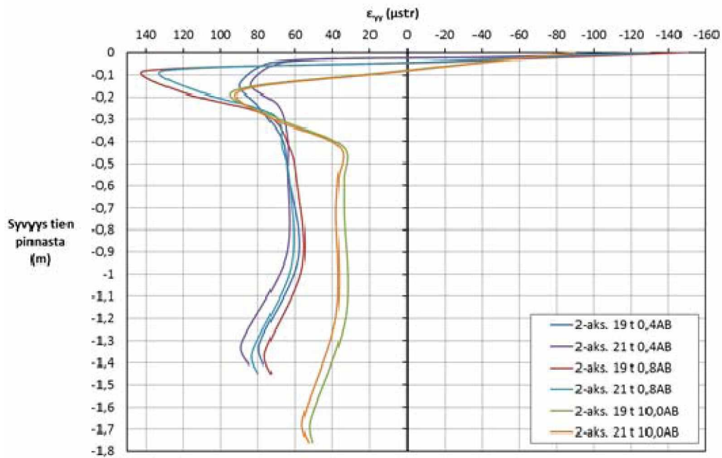
Vaakasuuntainen suhteellinen muodonmuutos \epsilon_{yy} 2-aks. 19 t & 21 t
