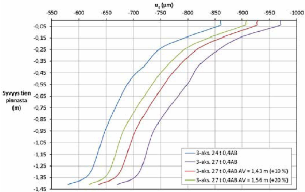
Pystysuuntainen hetkellinen siirtymä u_z , 3-aks., pidennetyn akselivälin vaikutus
