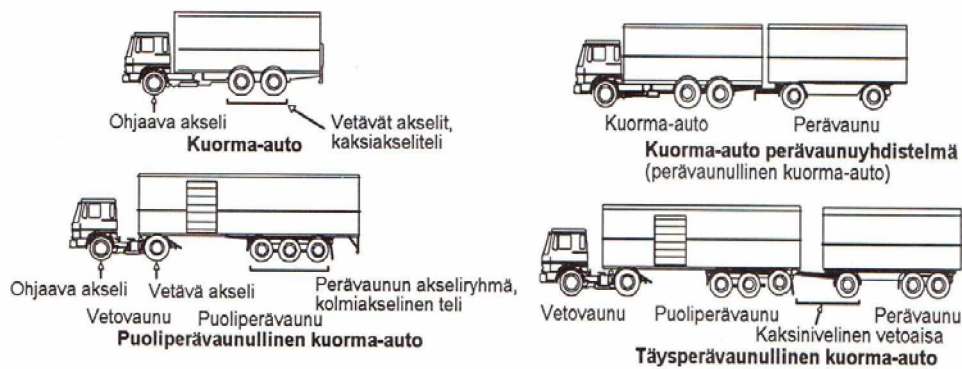
Kuva 6. Kuorma-autojen perustyyppit. (Mukaiituna Ehrola 1996, s. 33)
