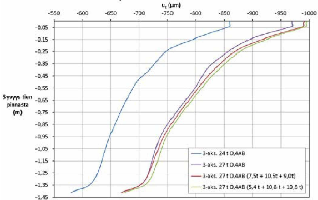
Pystysuuntainen hetkellinen siirtymä u_z , 3-aks., epätasaisesti jakautuneen kuorman vaikutus
