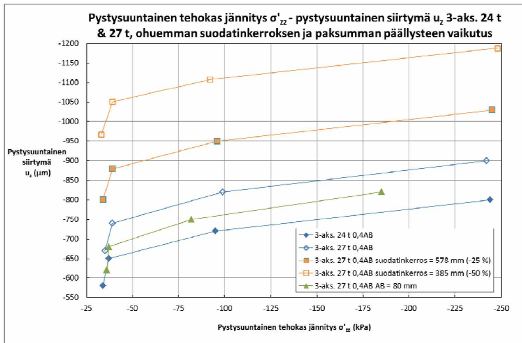
Kuva 87. Pystysuuntainen siirtymä pystysuuntaisen tehokkaan jännityksen funktiona 0,4AB-rakenteen sitomattomien kerrosten keskipisteissä sekä 100 mm syvyydellä pohjamaassa 3-akselisten telien tapauksissa – ohuemman suodatinkerroksen ja paksumman päällysteen vaikutus.
