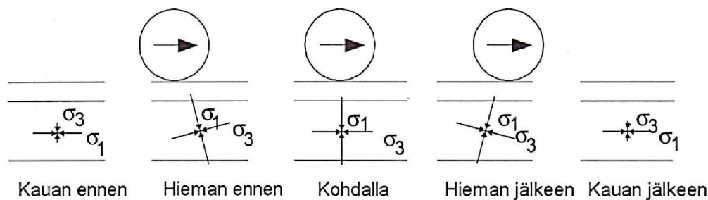
Kuva 20. Liikkuvan kuormituksen aiheuttama pääjännitysten kiertyminen. (Ehrola 1996, s. 290)
