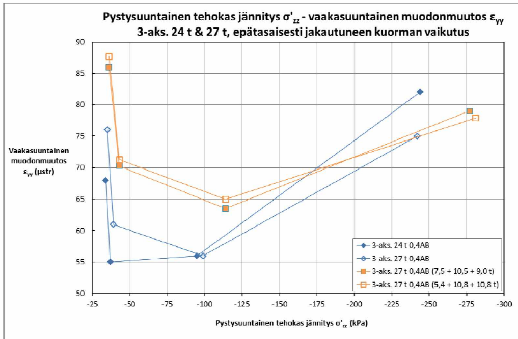
Kuva 80. Vaakasuuntainen muodonmuutos pystysuuntaisen tehokkaan jännityksen funktiona 0,4AB-rakenteen sitomattomien kerrosten keskipisteissä sekä 100 mm syvyydellä pohjamaassa 3-akselisten telien tapauksissa – epätasaisesti jakautuneen kuorman vaikutus.
