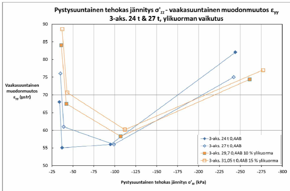
Kuva 78. Vaakasuuntainen muodonmuutos pystysuuntaisen tehokkaan jännityksen funktiona 0,4AB-rakenteen sitomattomien kerrosten keskipisteissä sekä 100 mm syvyydellä pohjamaassa 3-akselisten telien tapauksissa – ylikuorman vaikutus.
