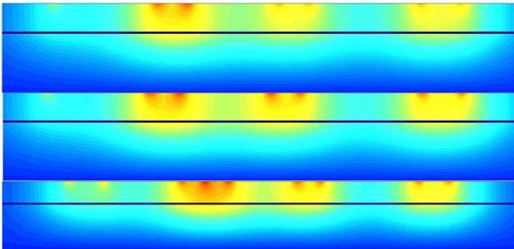
Kuva 71. Pystysuuntaisen hetkellisen siirtymän jakaumia 0,4AB-rakenteessa ja pohjamaassa. Ylhäällä 7-aks. 60 t, keskellä 7-aks. 64 t ja alhaalla 9-aks. 76 t.
