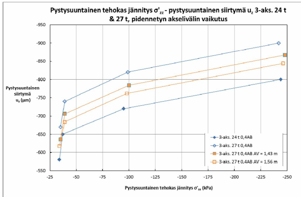
Kuva 81. Pystysuuntainen siirtymä pystysuuntaisen tehokkaan jännityksen funktiona 0,4AB-rakenteen sitomattomien kerrosten keskipisteissä sekä 100 mm syvyydellä pohjamaassa 3-akselisten teliin tapauksissa – pidennetyn akselivälin vaikutus.
