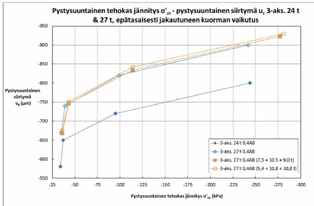
Kuva 79. Pystysuuntainen siirtymä pystysuuntaisen tehokkaan jännityksen funktiona 0,4AB-rakenteen sitomattomien kerrosten keskipisteissä sekä 100 mm syvyydellä pohjamaassa 3-akselisten teliin tapauksissa – epätasaisesti jakautuneen kuorman vaikutus.
