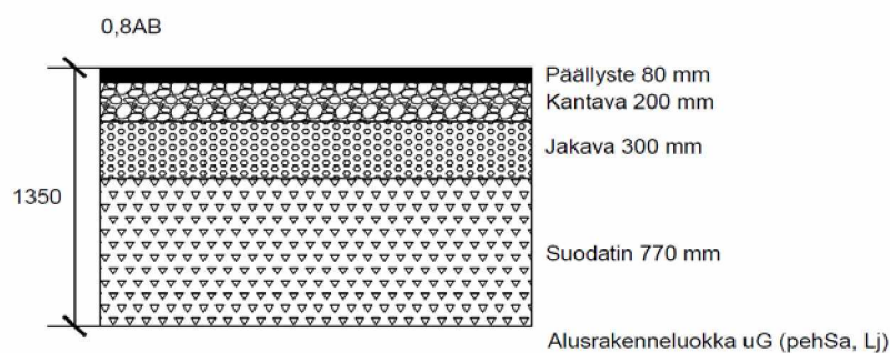
Kuva 62. Tarkasteltava tierakenne 0,8AB. (Tiehallinto 2004, s. 68)
