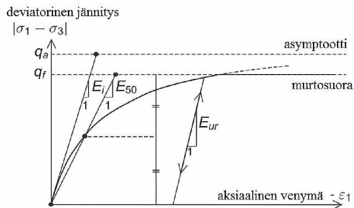
Kuva 60. Hardening soil -mallin hyperbolisen jännitys-muodonmuutoskäyttäytymisen periaate. (Mukailtuna Brinkgreve ym. 2011d, s. 51)
