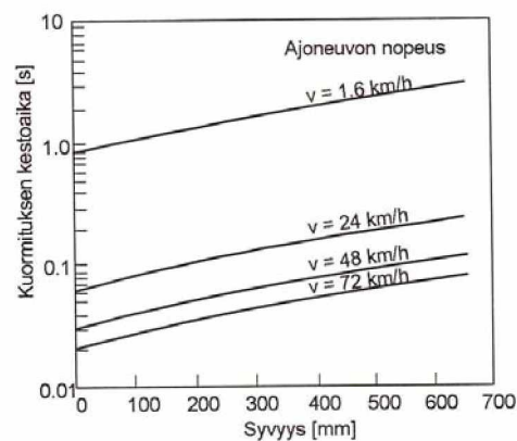
Kuva 15. Ajoneuvon nopeuden ja tarkastelusyvyuden vaikutus renkaan kuormitusaikaan tierakenteessa. (Ehrola 1996, s. 42)
