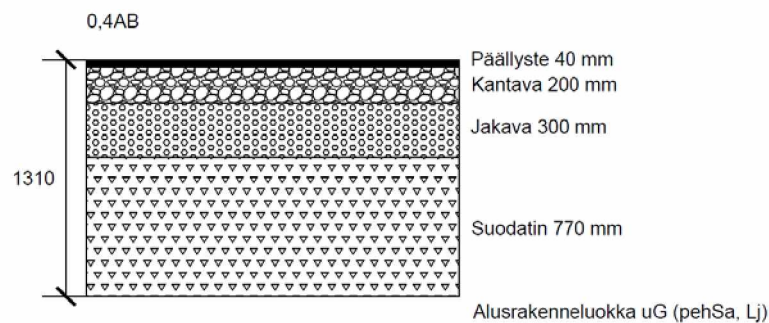
Kuva 61. Tarkasteltava tierakenne 0,4AB. (Mukailtuna Tiehallinto 2004, s. 29, 68)
