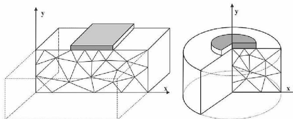
Kuva 56. Laskentatapavaihtoehdot Plaxis 2D:ssä: vasemmalla tasotapaus ja oikealla pyörähdyssymmetrinen tapaus. (Brinkgreve ym. 2011c, s. 17)
