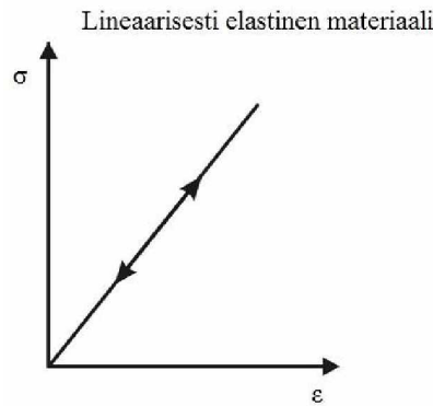
Kuva 59. Lineaarisesti elastisen materiaalin jännitys-muodonmuutoskäyttäytyminen. (Mukailtuna Korkiala-Tanttu 2008, s. 24)
