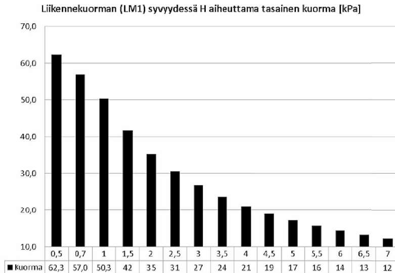
Kuva 54. Kuormakaavion LM1 aiheuttama tasainen kuorma syvyydellä H. Tarkoitettu vain eräiden geolujitettujen rakenteiden mitoittamiseen mitoitustavalla DA2*. (Liikennevirasto 2012, s. 40)
