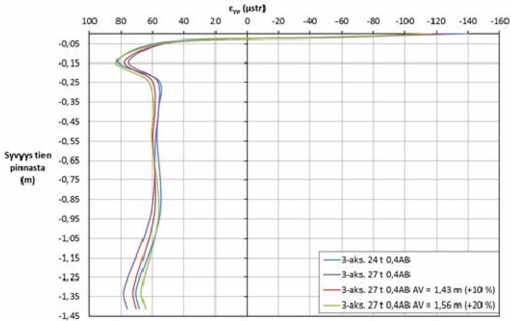
Vaakasuuntainen suhteellinen muodonmuutos \epsilon_{yy} 3-aks., pidennetyn akselivälin vaikutus
