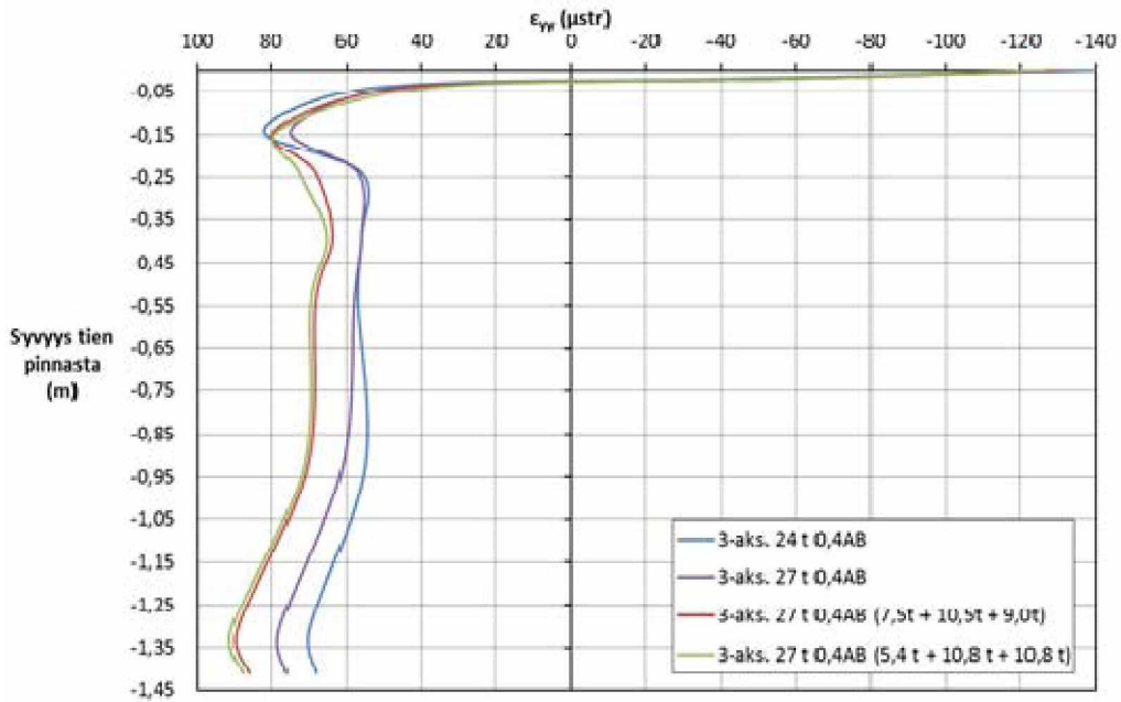
Vaakasuuntainen suhteellinen muodonmuutos \epsilon_{yy} , 3-aks., epätasaisesti jakautuneen kuorman vaikutus
