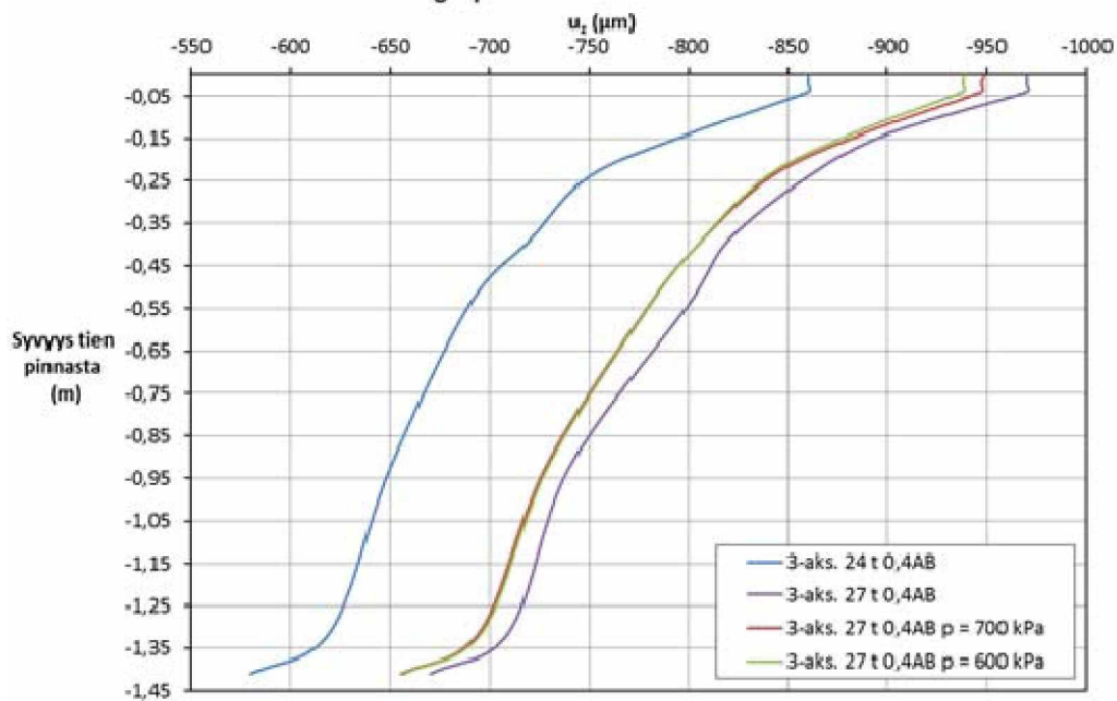
Pystysuuntainen hetkellinen siirtymä u_z , 3-aks., alennettujen rengaspaineiden vaikutus
