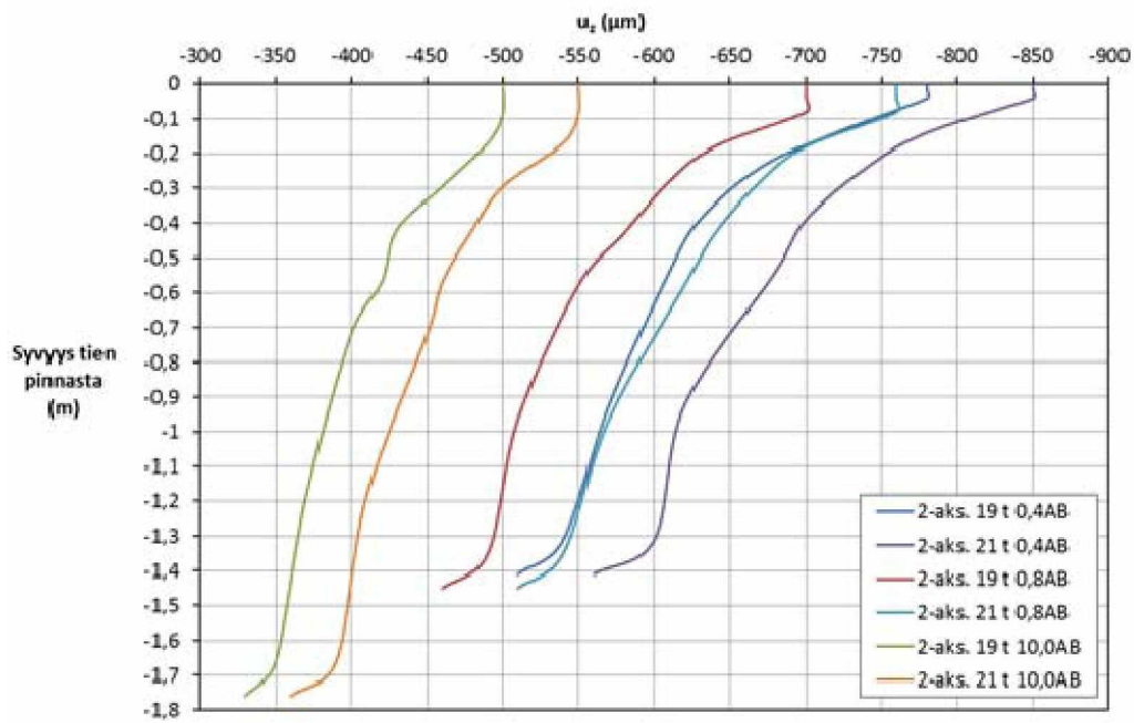
Pystysuuntainen hetkellinen siirtymä u_z , 2-aks. 19 t & 21 t
