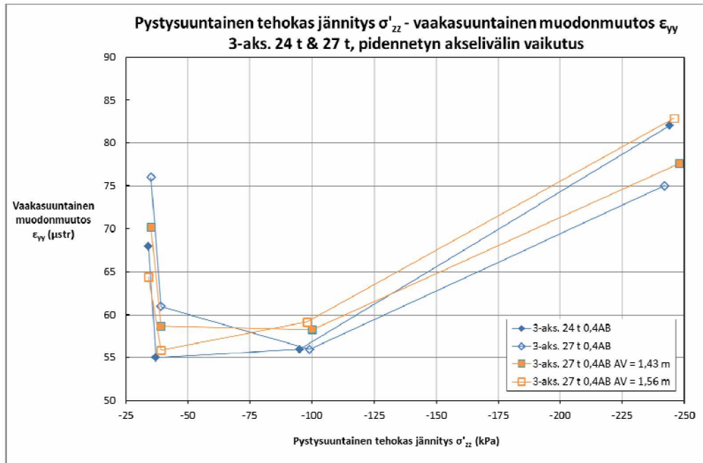
Kuva 82. Vaakasuuntainen muodonmuutos pystysuuntaisen tehokkaan jännityksen funktiona 0,4AB-rakenteen sitomattomien kerrosten keskipisteissä sekä 100 mm syvyydellä pohjamaassa 3-akselisten telien tapauksissa – pidennetyn akselivälin vaikutus.
