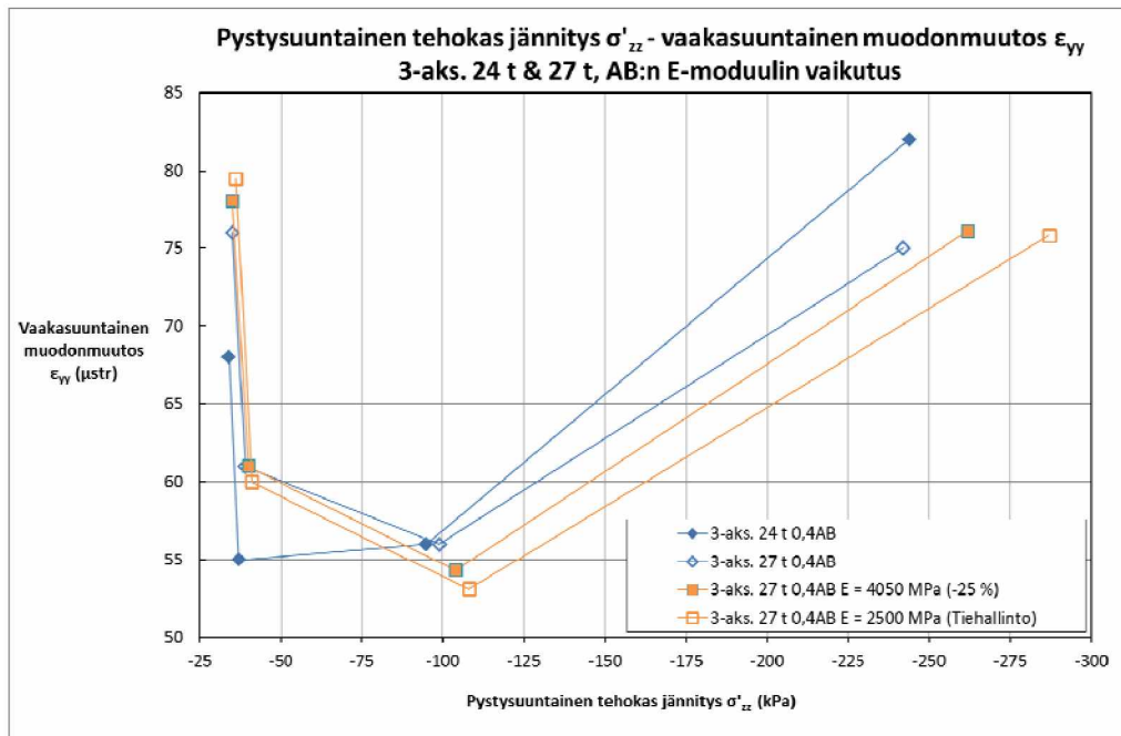
Kuva 86. Vaakasuuntainen muodonmuutos pystysuuntaisen tehokkaan jännityksen funktiona 0,4AB-rakenteen sitomattomien kerrosten keskipisteissä sekä 100 mm syvyydellä pohjamaassa 3-akselisten telien tapauksissa – AB:n E-moduulin vaikutus.
