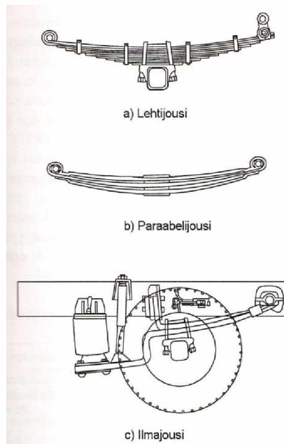
Kuva 10. Kuorma-autojen tyypillisimmät jousitustyyppit. (Ehrola 1996, s. 71)
