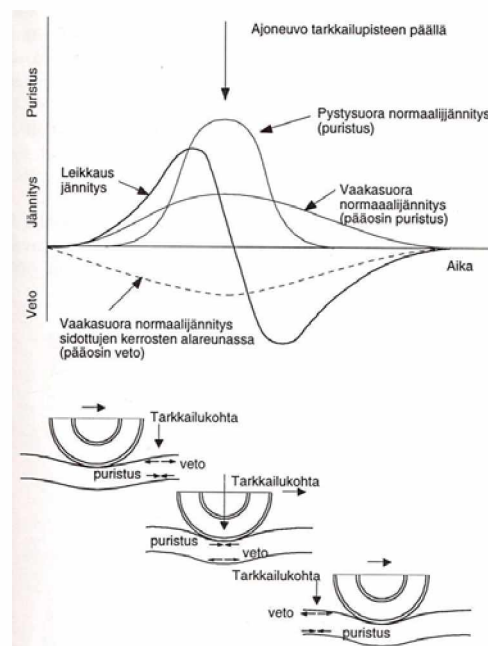
Kuva 19. Normaalijännitys- ja leikkausjännitykset tierakenteessa ajoneuvon renkaan lähestyessä ja ylittäessä tarkastelukohtaa. (Ehrola 1996, s. 41)
