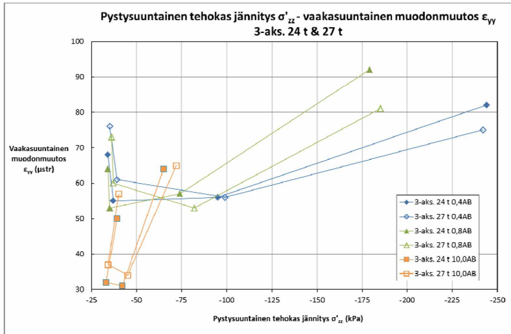
Kuva 76. Vaakasuuntainen muodonmuutos pystysuuntaisen tehokkaan jännityksen funktiona 0,4AB, 0,8AB ja 10,0AB-rakenteiden sitomattomien kerrostien keskipisteissä sekä 100 mm syvyydellä pohjamaassa 3-akselisten 24 ja 27 tonnin telien tapauksissa.
