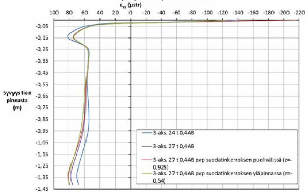
Vaakasuuntainen suhteellinen muodonmuutos \epsilon_{yy} 3-aks., korkeamman pohjavedenpinnan vaikutus
