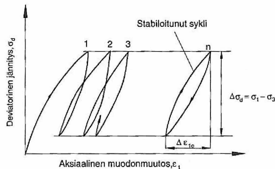
Kuva 32. Sitomattoman materiaalin kuormitus-muodonmuutoskäyttäytyminen syklisessä kuormituksessa. (Ehrola 1996, s. 173)
