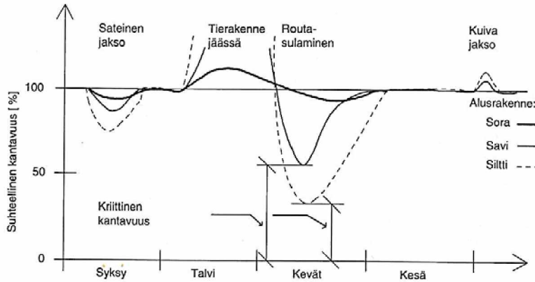
Kuva 38. Tierakenteen kantavuuden vuodenaikaisvaihtelu erilaisilla alusrakenteilla. (Ehrola 1996, s. 125)
