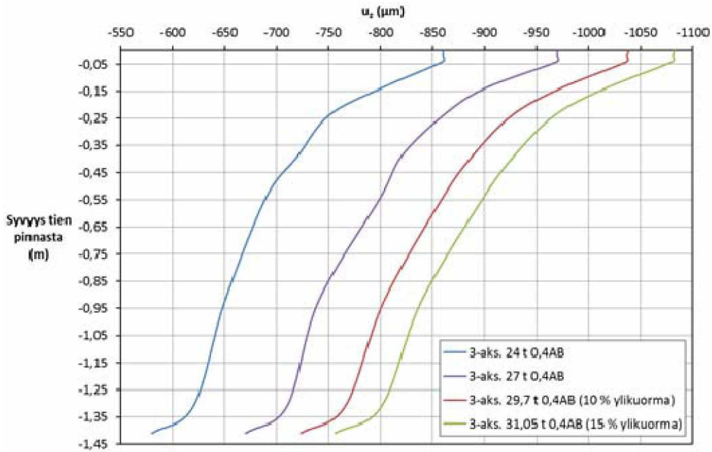
Pystysuuntainen hetkellinen siirtymä u_z , 3-aks., ylikuorman vaikutus
