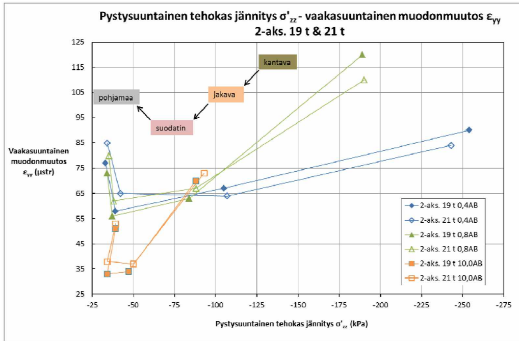
Kuva 74. Vaakasuuntainen muodonmuutos pystysuuntaisen tehokkaan jännityksen funktiona 0,4AB, 0,8AB ja 10,0AB-rakenteiden sitomattomien kerrostojen keskipisteissä sekä 100 mm syvyydellä pohjamaassa 2-akselisten 19 ja 21 tonnin telien tapauksissa.
