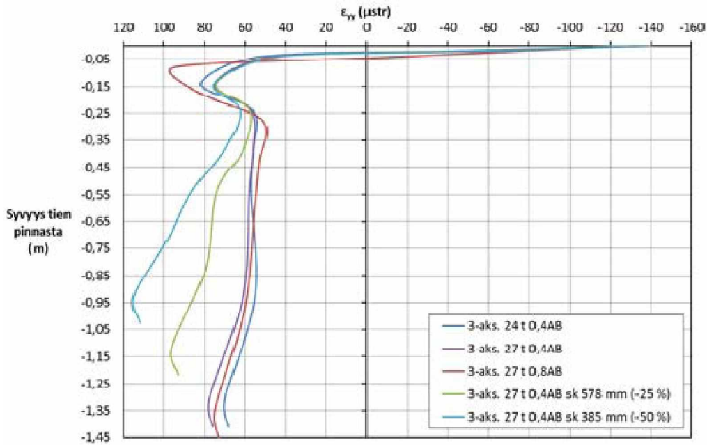
Vaakasuuntainen suhteellinen muodonmuutos \epsilon_{yy} 3-aks., paksumman AB:n ja ohuemman suodatinkerroksen vaikutus
