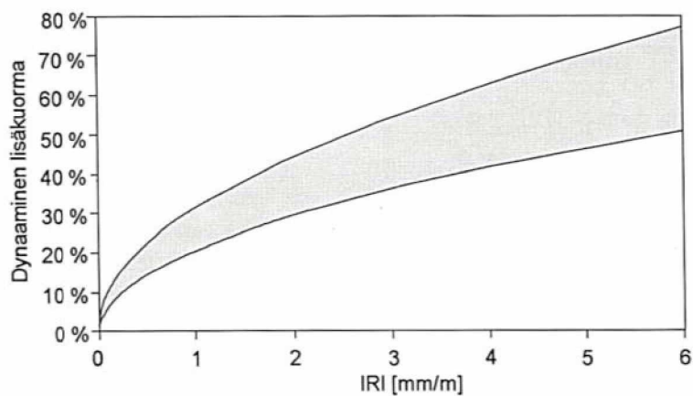
Kuva 2. Tienpinnan epätasaisuuden vaikutus kuorma-auton dynaamisten maksimilisäkuormien suuruuteen. (Ehrola 1996, s. 70)
