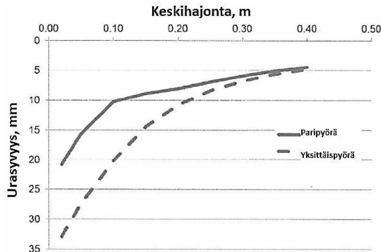
Kuva 5. Päällystekerroksen urasyvyyden riippuvuus raskaiden ajoneuvojen ajolinjojen keskihajonnasta. (Mukaiituna Said & Hakim 2013, s. 33)
