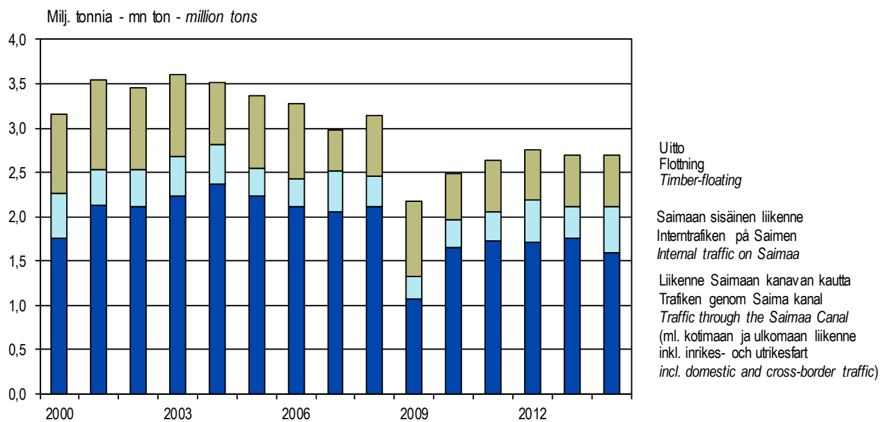
Figure 14. Goods traffic in Vuoksi watercourse (Saimaa) total, 2000-2014
