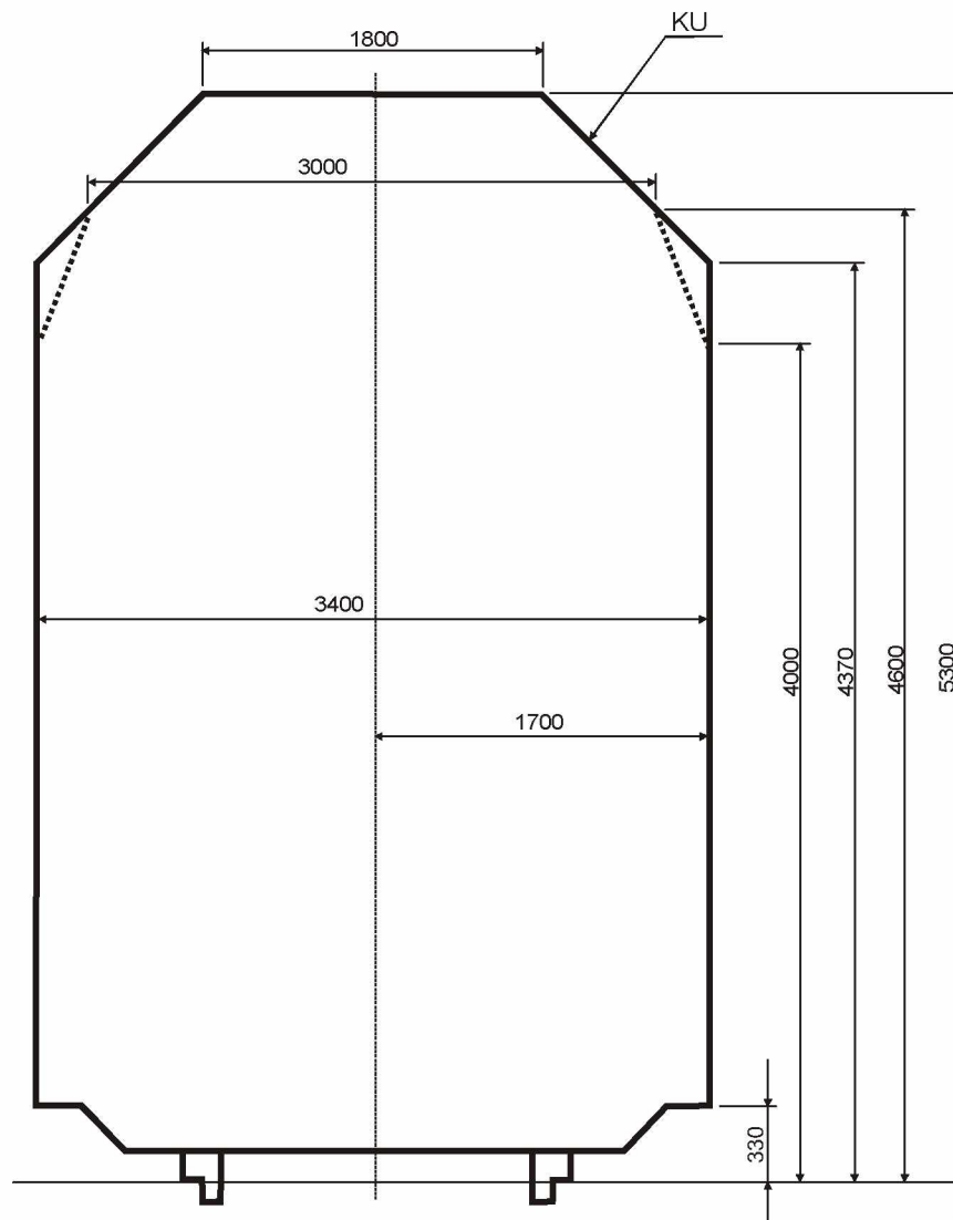
Kuva 10. Kuormaulottuma.
