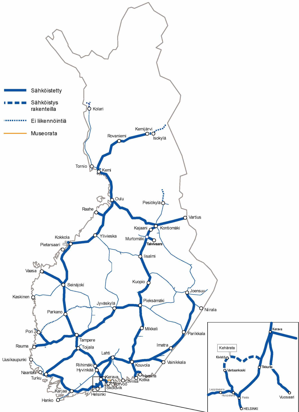
Kuva 6. Sähköistetyt radat
