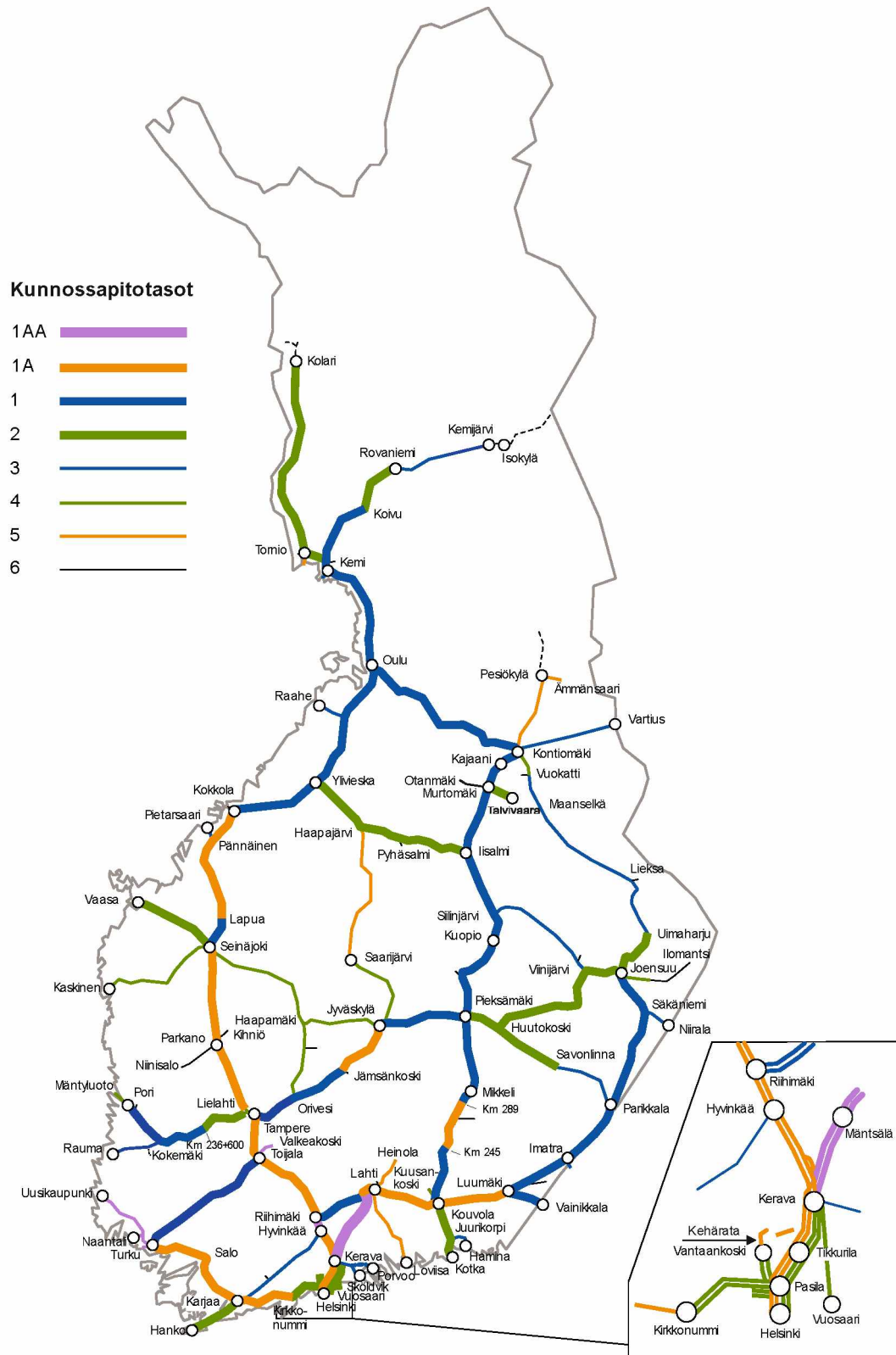
Kuva 2. Pääratojen kunnossapitotasot
