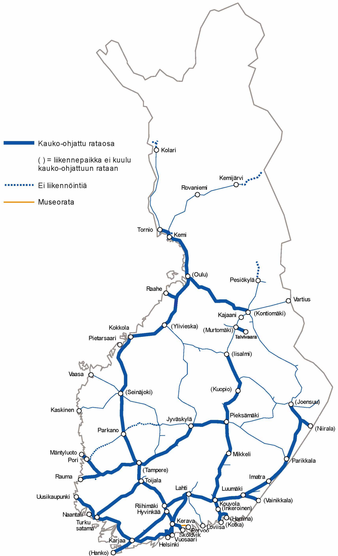
Kuva 5. Kauko-ohjatut radat
