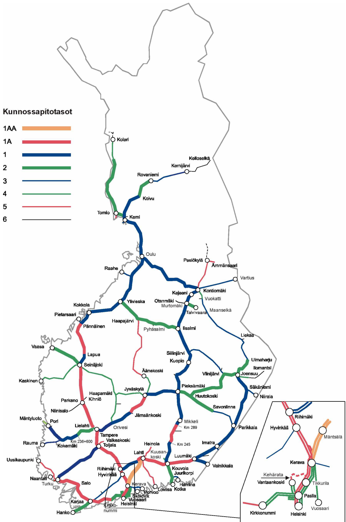
Kuva 2. Pääratojen kunnossapitotasot
