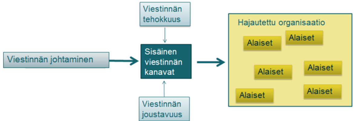
Kuva 1. Tutkielman viitekehys
