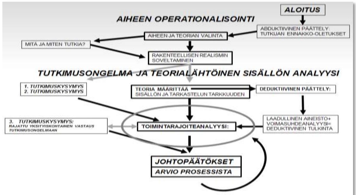
Kuva1. Tutkimusprosessi
